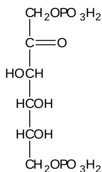
Fructosa 1 - 6 difosfato
