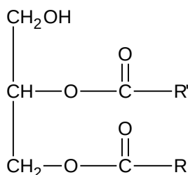
DAG
