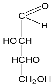
Treosa
