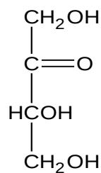
Eritrosa
