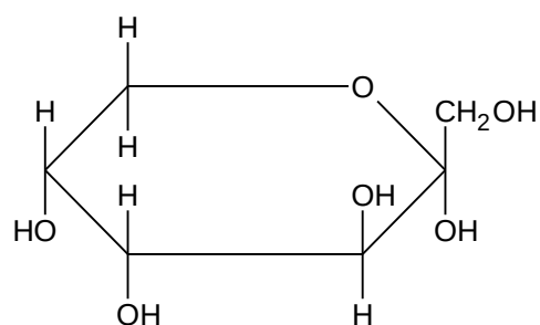
\alpha - Fructopiranosa
