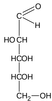
Arabinosa
