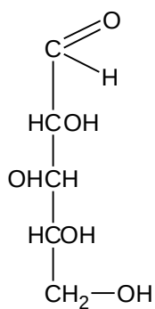
Xilosa
