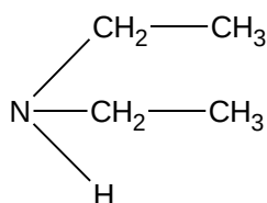
amina secundaria
