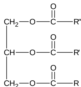
TAG
