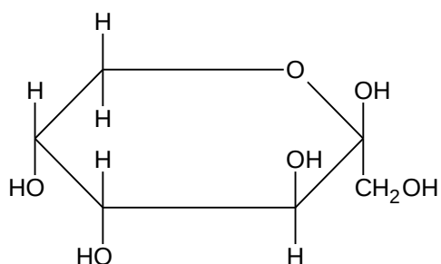
\beta - Fructopiranosa
