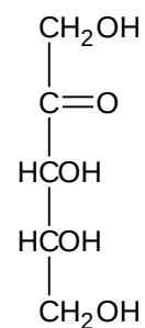
Ribulosa
