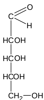
Ribosa
