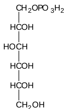
Glucosa 1 fosfato
