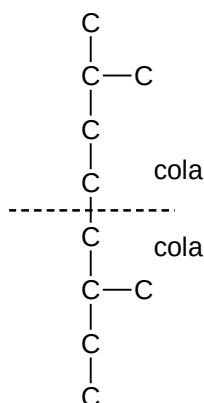
Irregularmente
