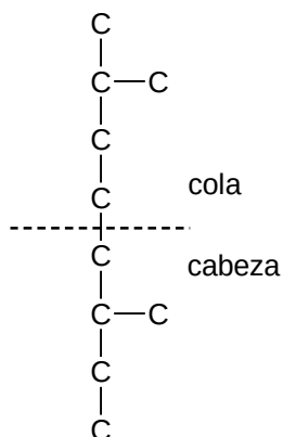
Regularmente
