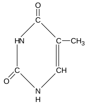
Timina
