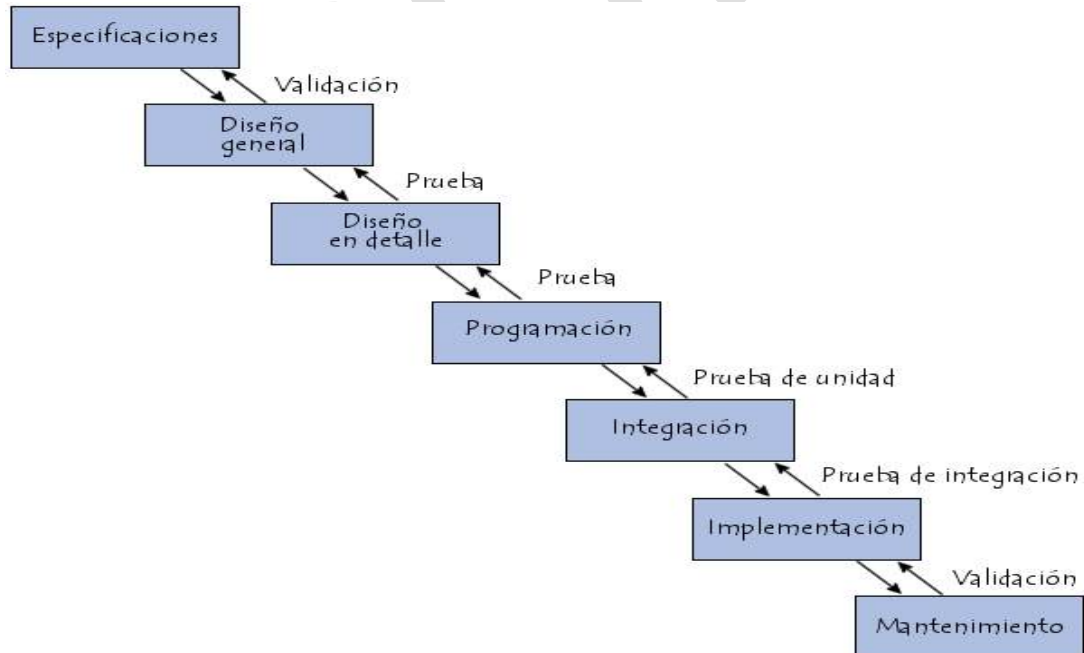
Figura 16: Modelo cascada
