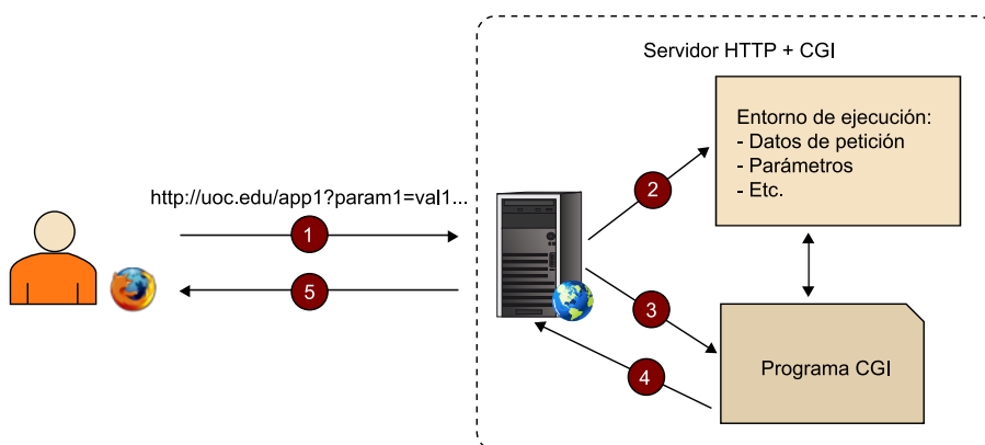
Figura 4. Funcionamiento básico de un CGI
