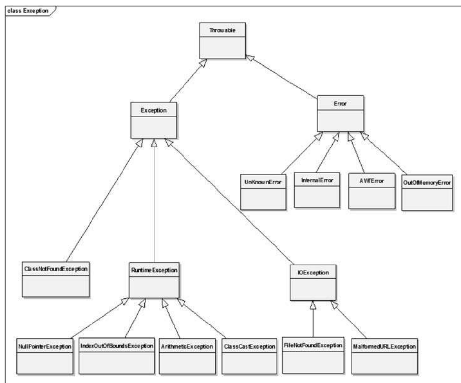
Figura 2. Jerarquía simplificada de clases derivadas de Throwable
