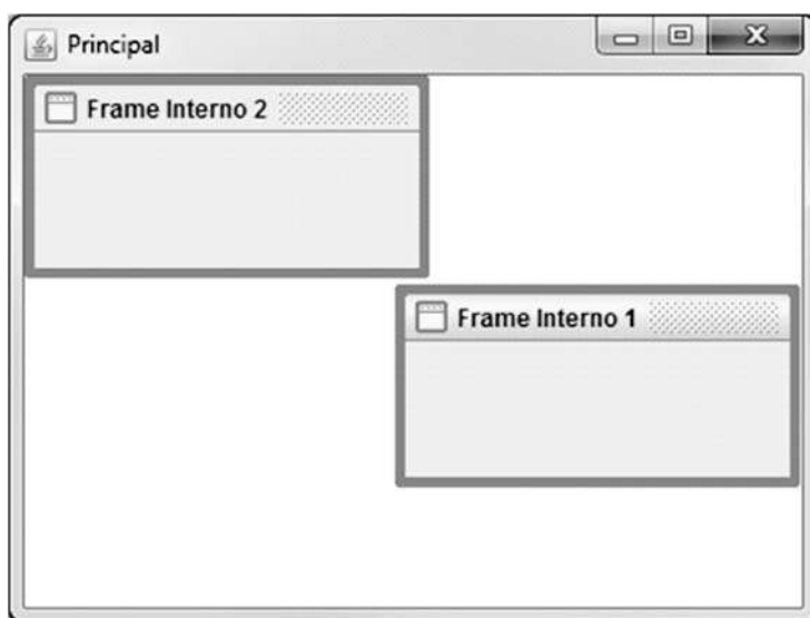
Figura 22. JInternalFrame
