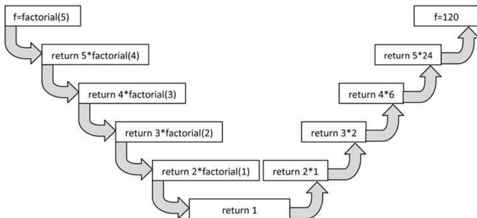
Figura 1. Representación de funcionamiento de recursividad
