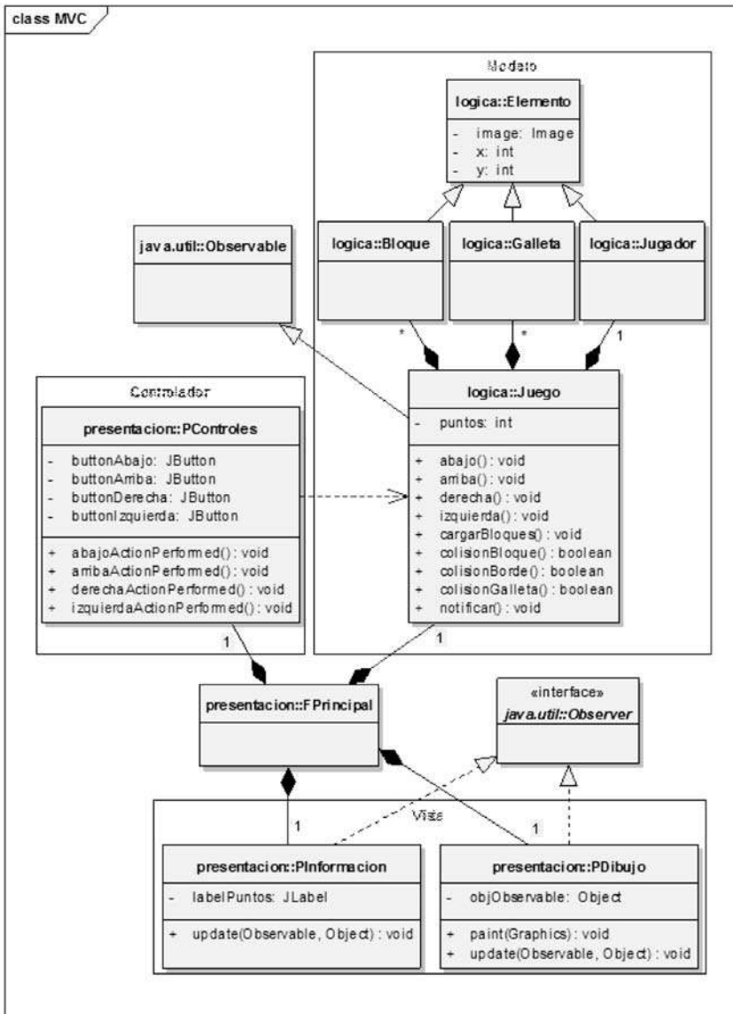
Figura 85. Diagrama de clases del juego Pacman basado en MVC
