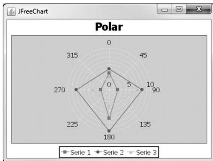
Figura 78. Polar Chart
