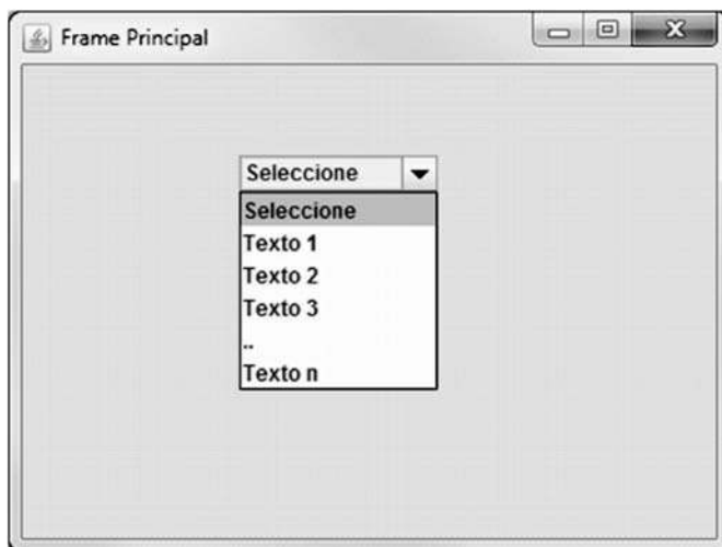
Figura 26. JComboBox
