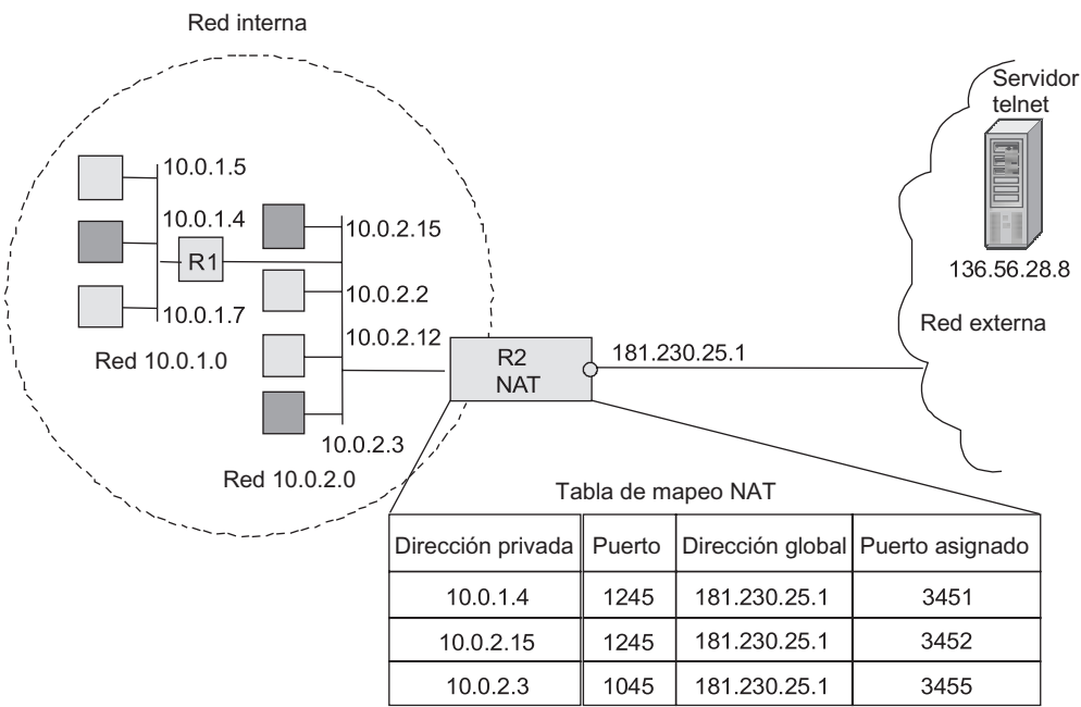
FIGURA 20.9 NAT: traducción de dirección y número de puerto para sesiones salientes TCP/UDP.
