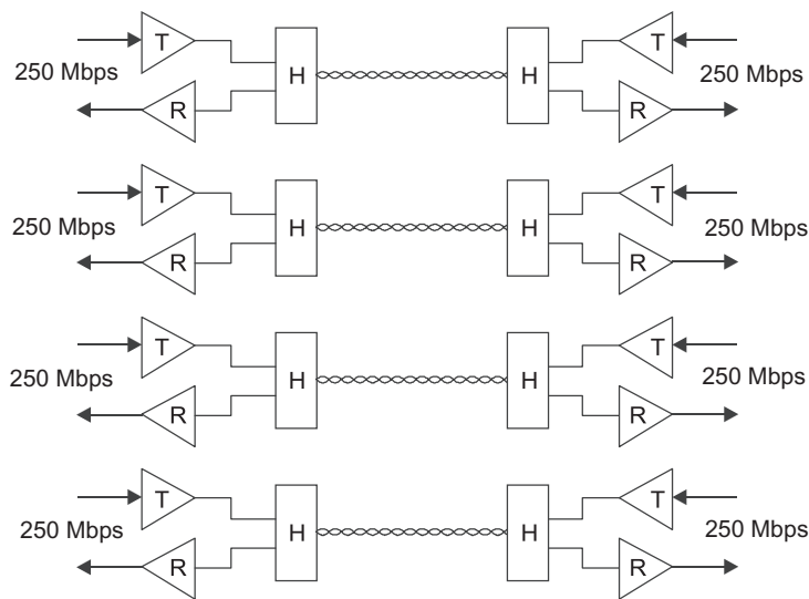
FIGURA 13.7 Transmisión bidireccional utilizando cuatro UTP de categoría 5.
