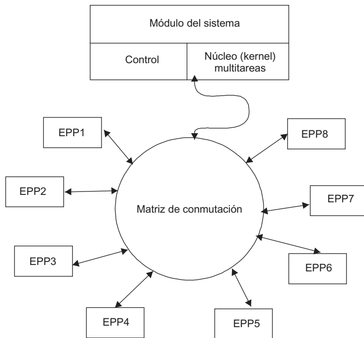
FIGURA 15.9 Diseño estructural del switch EtherSwitch sugerido por Kalpana.
