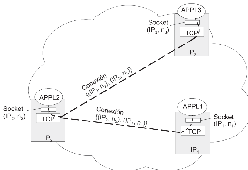
FIGURA 19.6 Un socket puede participar en varias conexiones.
