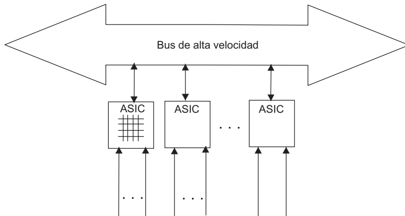
FIGURA 15.18 Arquitectura de un switch combinado basada en una matriz de conmutación y un bus común.
