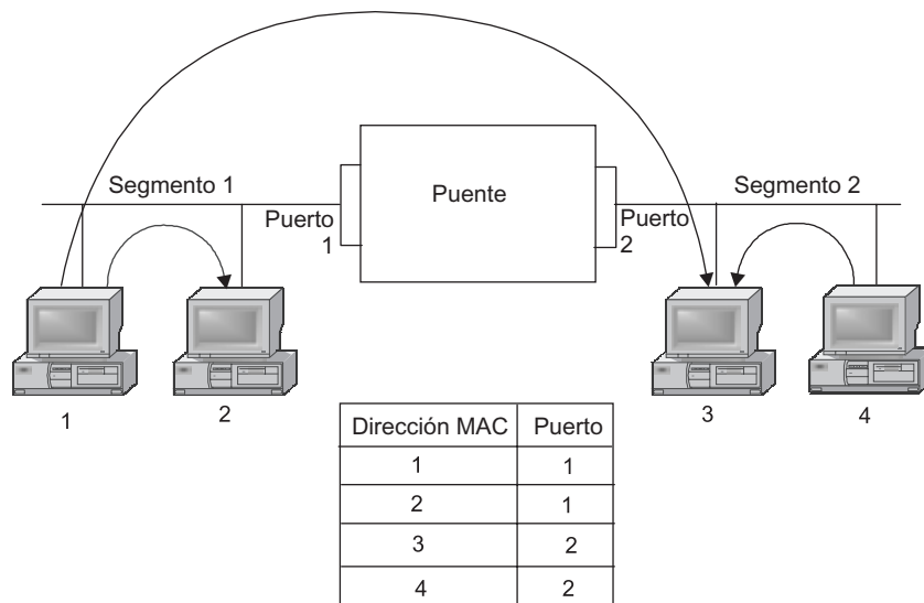
FIGURA 15.4 Principio de operación de un switch o puente transparente.
