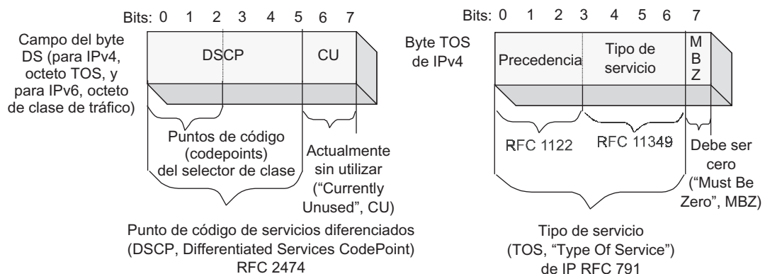
FIGURA 20.5 Correspondencia de los campos del byte DS con los campos de los bytes TOS.
