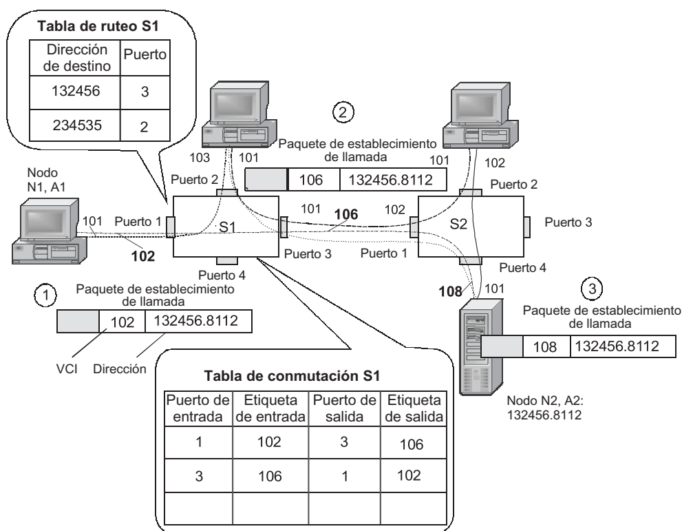
FIGURA 21.1 Establecimiento de un circuito virtual
