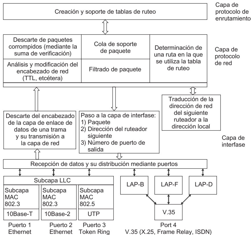
FIGURA 20.10 Modelo funcional de un router.
