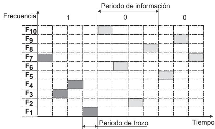
FIGURA 10.13 Relación entre la velocidad de la información y la velocidad de trozos.
