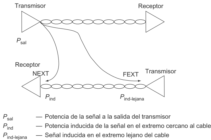
FIGURA 8.10 Atenuación transitoria.
