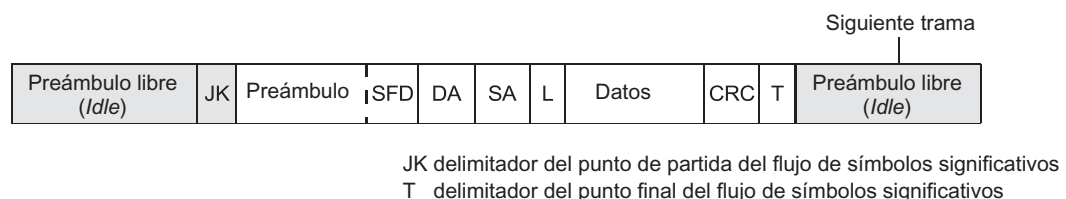
FIGURA 13.3 Flujo continuo de datos en 100Base-FX/TX.
