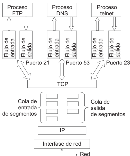
FIGURA 19.4 Formación de segmentos TCP de un flujo no estructurado de bytes.
