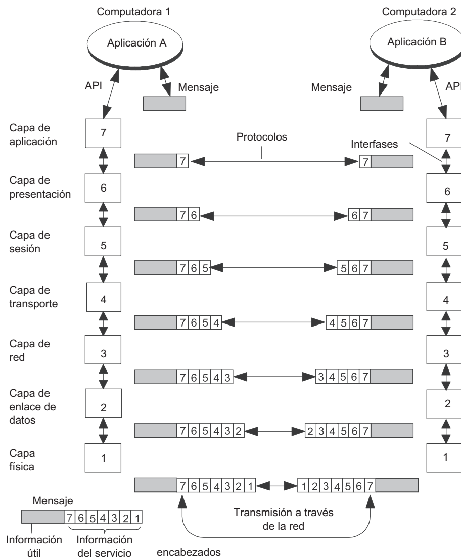
FIGURA 4.6 Modelo ISO/OSI.
