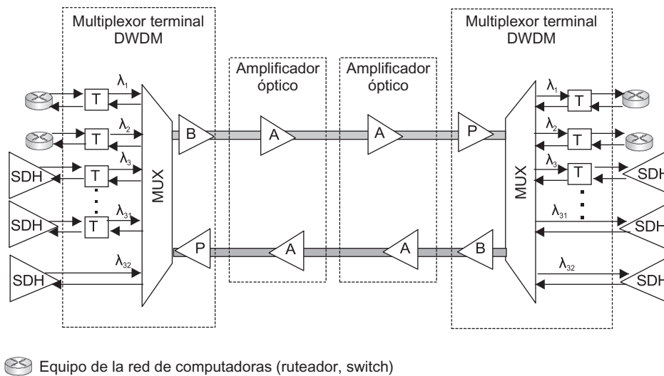
FIGURA 11.14 Troncal punto a punto de ultralarga distancia basada en multiplexores terminales DWDM.
