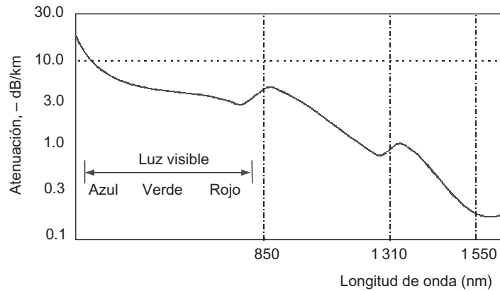
FIGURA 8.9 Ventanas de transparencia de la fibra óptica.
