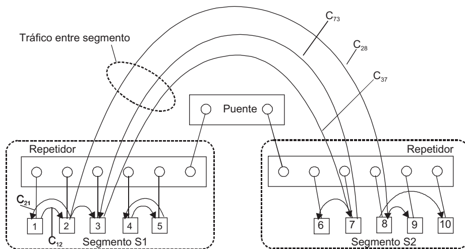
FIGURA 15.3 Cambio de la red después de la segmentación.
