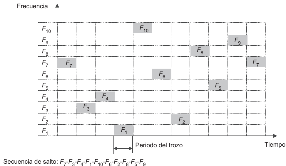
FIGURA 10.12 Dispersión del salto de frecuencias.
