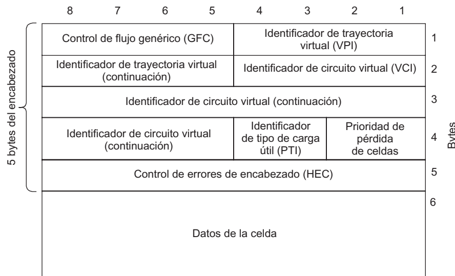
FIGURA 21.11 Formato de celda ATM.
