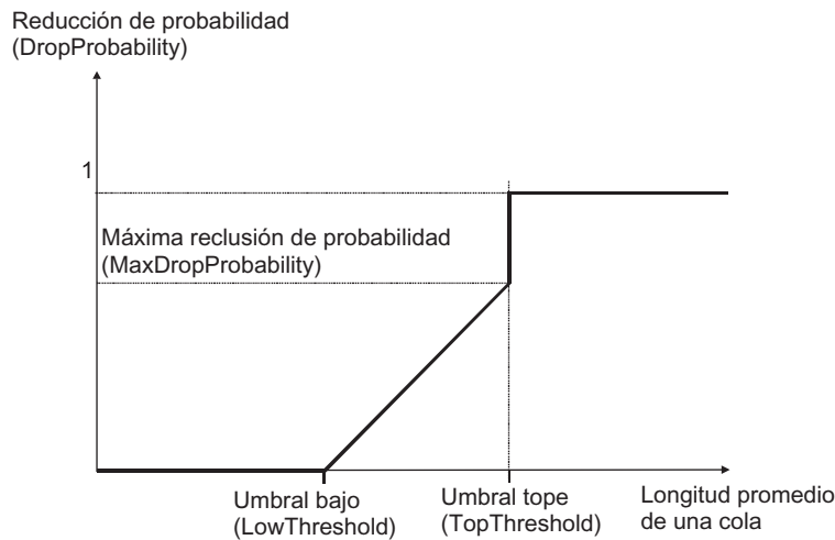
FIGURA 20.2 Probabilidad de descartar de paquetes en los que se utiliza el algoritmo RED.
