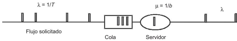
FIGURA 7.3 Modelo M/M/1.
