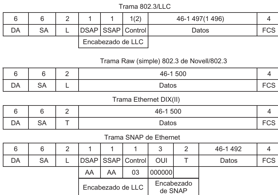
FIGURA 12.9 Formatos de las tramas de Ethernet.
