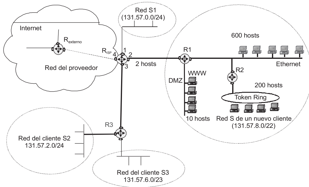
FIGURA 18.18 Elaboración de superredes ( supernetting ).
