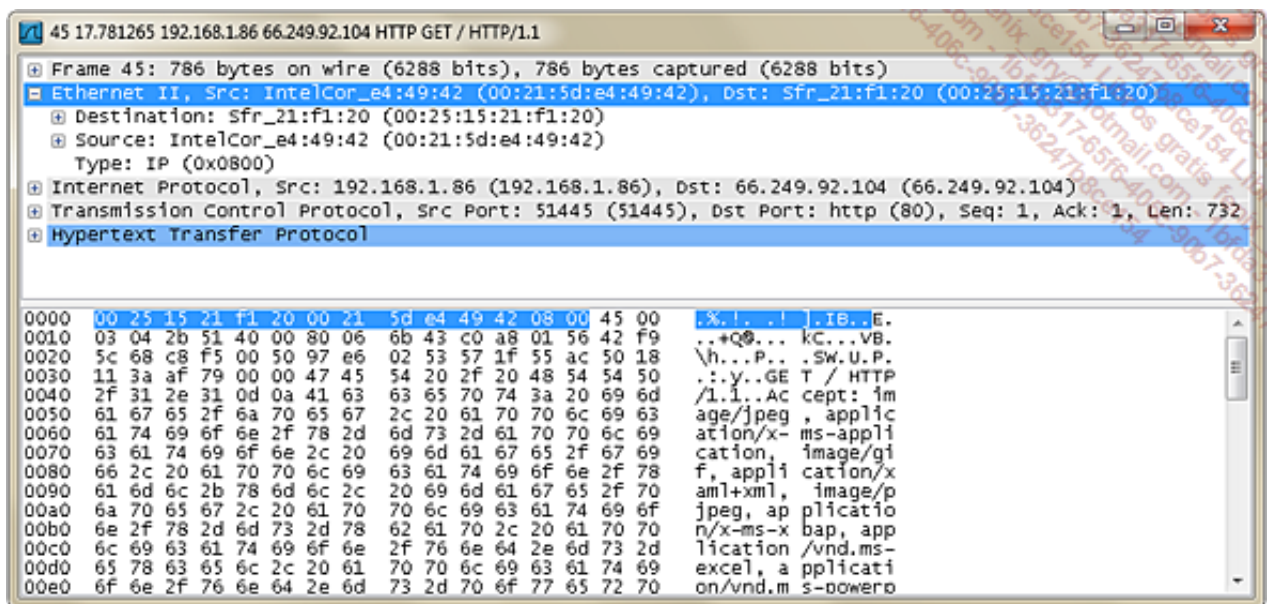
Ejemplo de trama HTTP capturada
