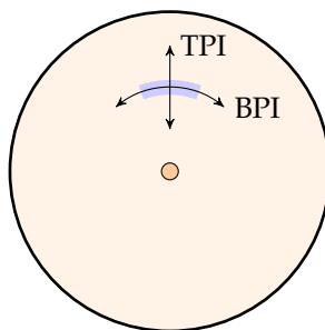
Figura 4.15: Definición de las unidades de densidad de almacenamiento
