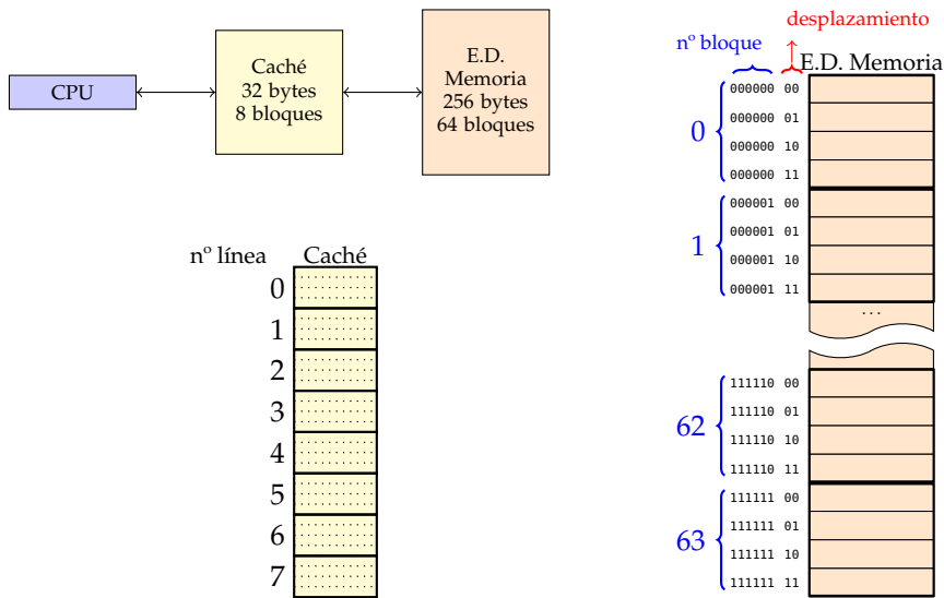
Figura 3.4: Espacio de direcciones de memoria y organización en líneas de la memoria caché
