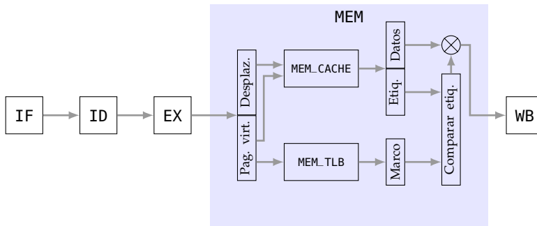
Figura 3.57: Caché indexada virtualmente y etiquetada físicamente (V/P)
