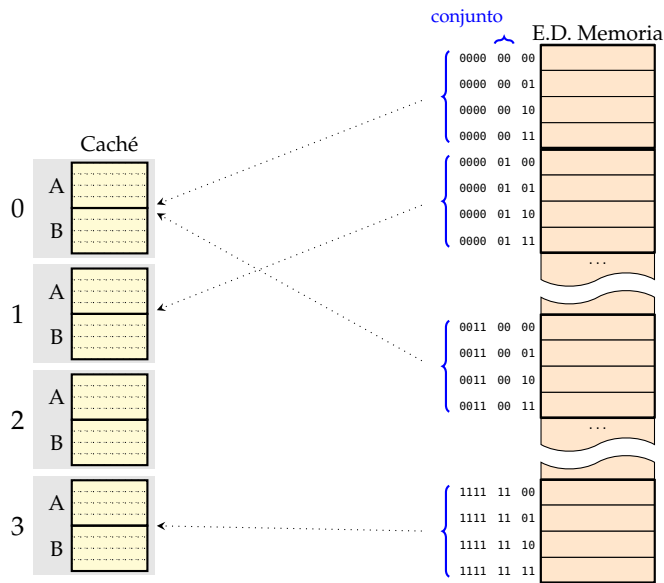
Figura 3.21: Asignación de bloques dentro de una memoria caché asociativa por conjuntos
