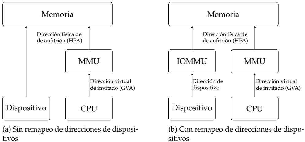
Figura 4.18: Estrategias de remapeo de dispositivos DMA
