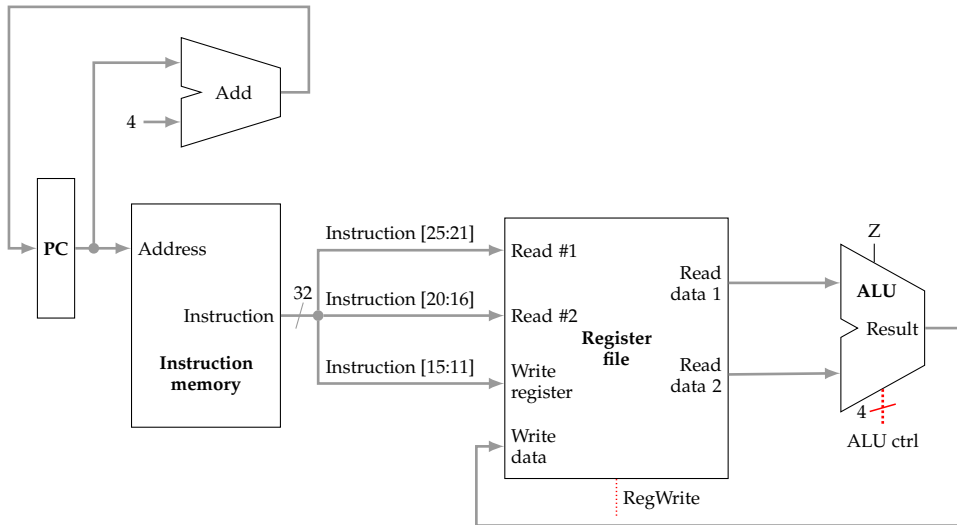
Figura 2.10: Camino de datos para la ejecución de instrucciones de tipo R (instrucciones lógicas y aritméticas sobre enteros)
