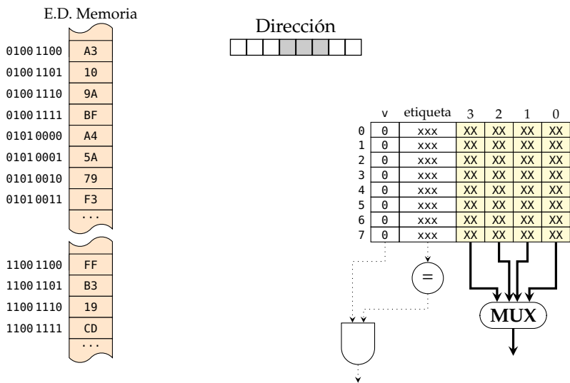
Figura 3.8: Correspondencia directa: situación inicial con la caché vacía
