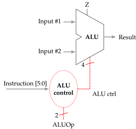
Figura B.1: Unidad de control de la ALU
