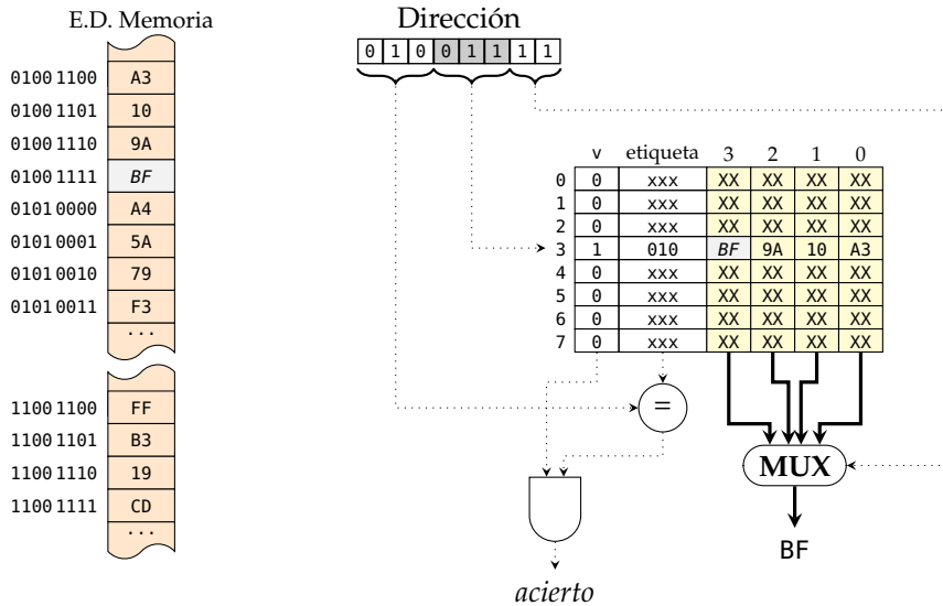
Figura 3.11: Correspondencia directa: petición de lectura de un byte sobre la dirección 4Fh, que produce un acierto de caché
