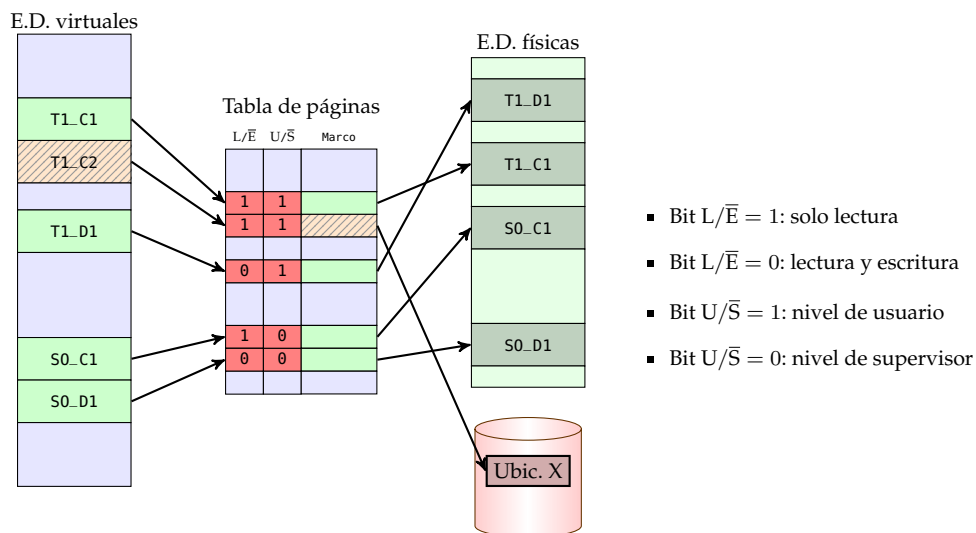
Figura 3.48: Bits de protección asociados a las páginas de una tarea y del sistema operativo
