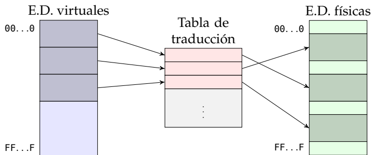
Figura 3.41: Traducción por bloques de las direcciones virtuales a direcciones físicas
