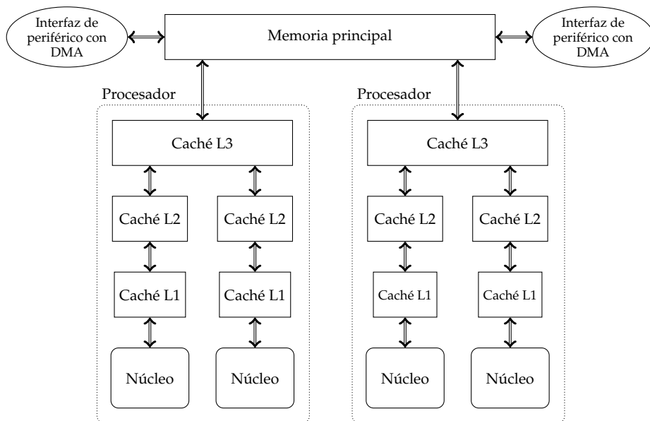
Figura 3.35: Ejemplo de multiprocesador con múltiples núcleos por procesador y varios niveles de caché
