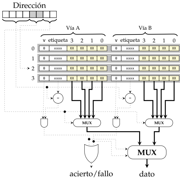
Figura 3.22: Estructura de una caché asociativa por conjuntos
