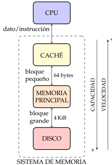
Figura 3.37: Jerarquía de memoria de tres niveles
