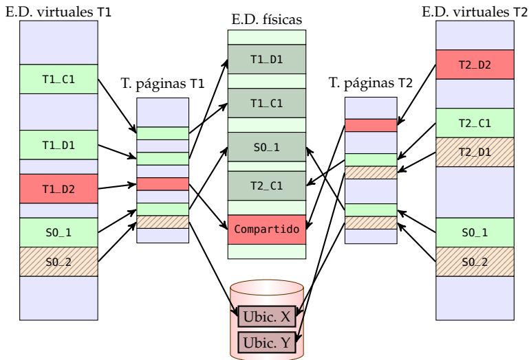
Figura 3.49: Compartición de una página de memoria entre dos tareas
