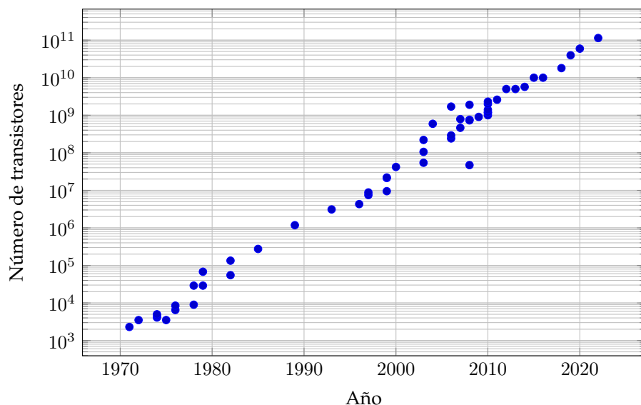
Figura 2.57: Número de transistores en los procesadores en las últimas décadas
