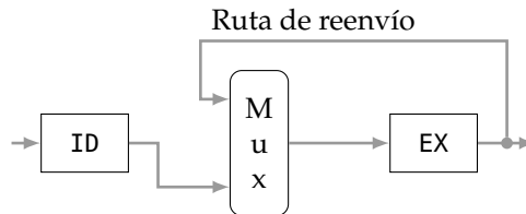
Figura 2.35: Implementación de la ruta de reenvío Salida EX → Entrada EX
