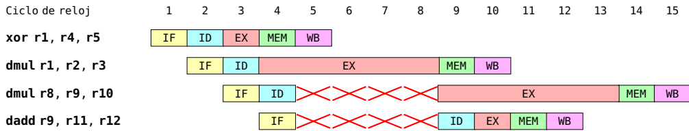
Figura 2.28: Ejecución de operaciones multiciclo no segmentadas
