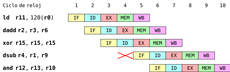
Figura 2.21: Ejecución segmentada asumiendo una única memoria
