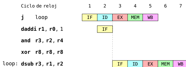
Figura 2.24: Ejecución segmentada con una detención por riesgo de control en un salto incondicional
