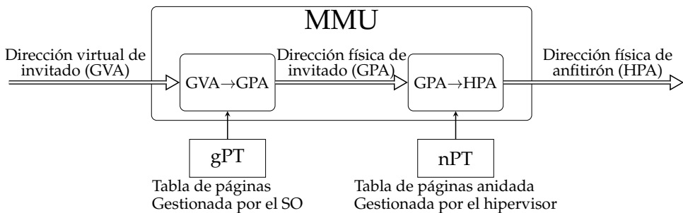
Figura 3.61: Traducción empleando paginación anidada
