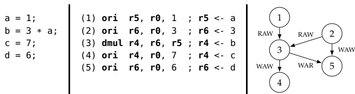
Figura 2.42: Ejemplo de dependencias producidas por el reciclaje de registros por parte del compilador
