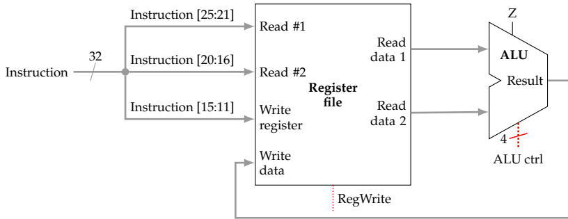
Figura 2.9: Ejecución de instrucciones de tipo R
