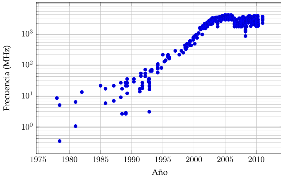
Figura 2.58: Frecuencia de los procesadores Intel en las últimas décadas
