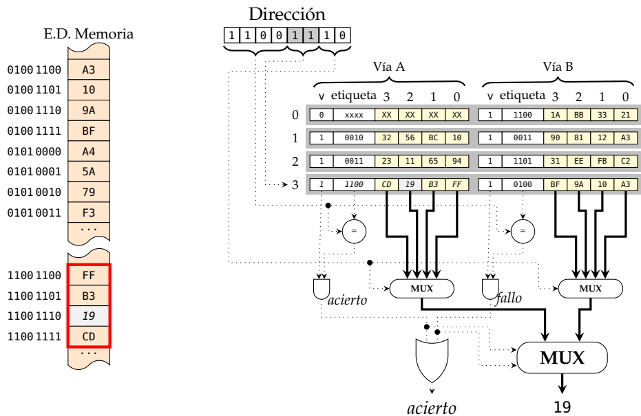
Figura 3.25: Correspondencia asociativa por conjuntos: reemplazo del bloque en la vía A del conjunto 3 y la caché sirve el byte solicitado
