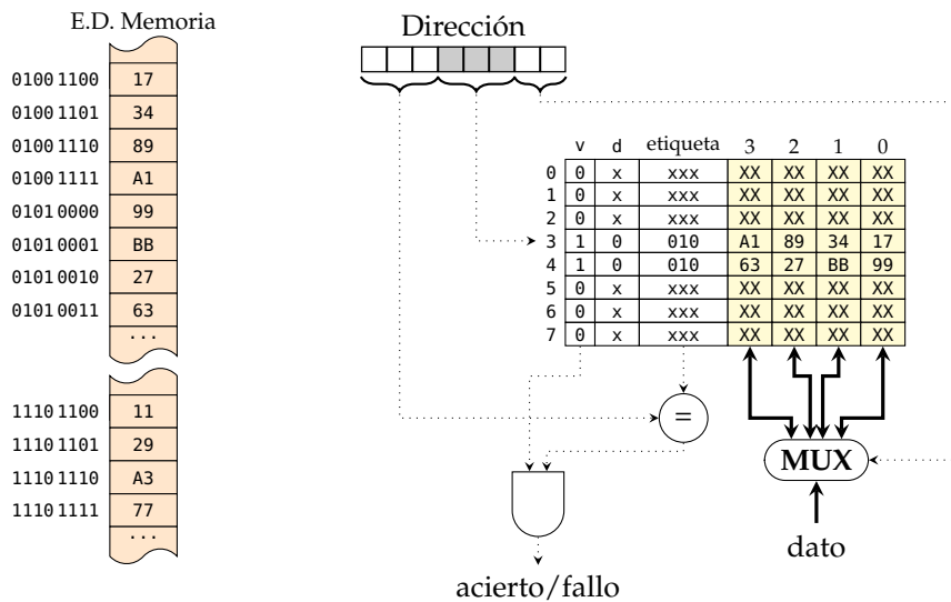
Figura 3.26: Funcionamiento de la estrategia de escritura write-back : situación inicial de la caché y del espacio de direcciones de memoria
