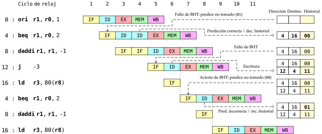
Figura 2.52: Funcionamiento del predictor de saltos de 2 bits
