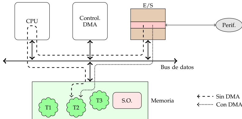
Figura 4.6: Movimiento de datos durante una operación de entrada sin DMA y con DMA en presencia de un sistema operativo multitarea
