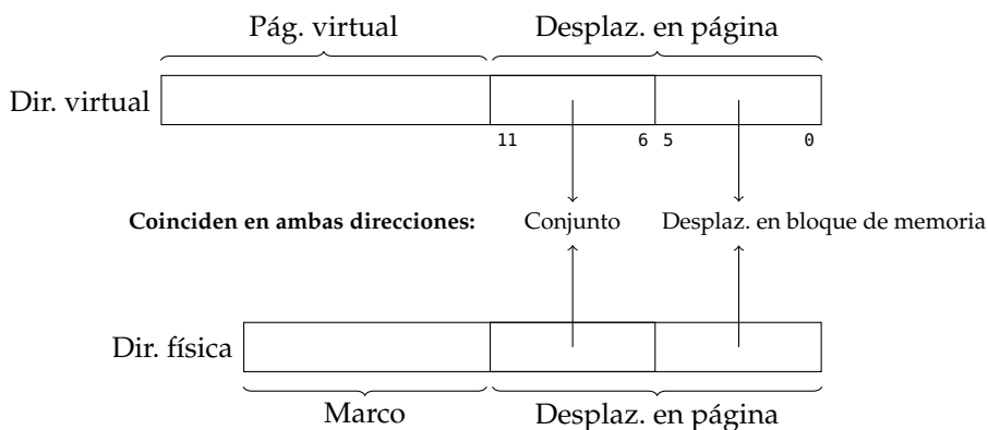
Figura 3.58: Obtención del conjunto de caché a partir del desplazamiento de la dirección física
