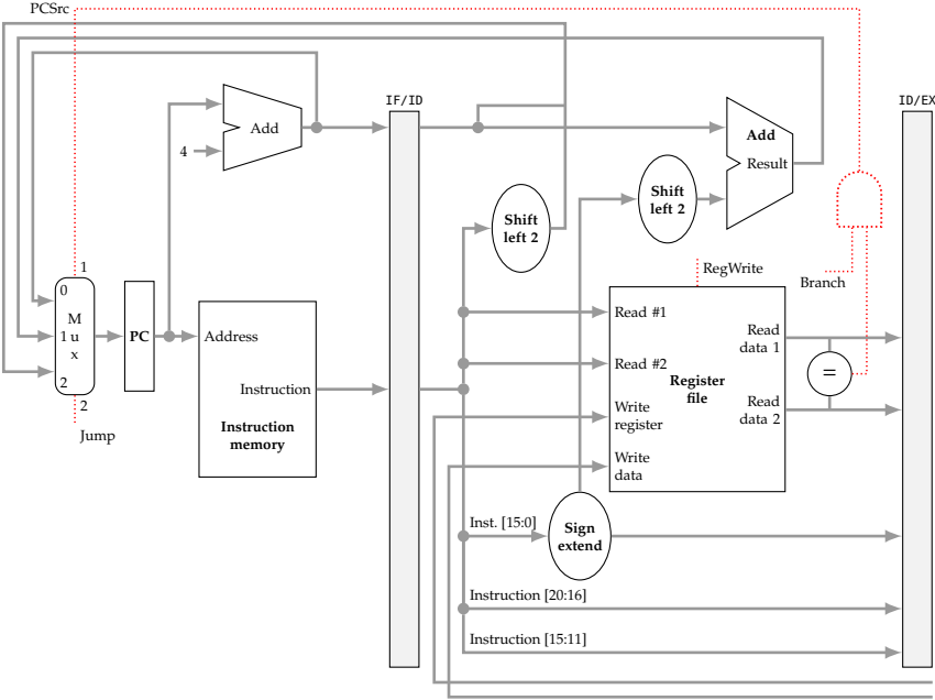
Figura 2.47: Etapas IF e ID para la evaluación agresiva del salto beq
