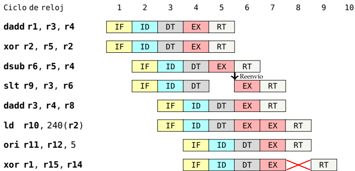
Figura 2.56: Ejecución superescalares
