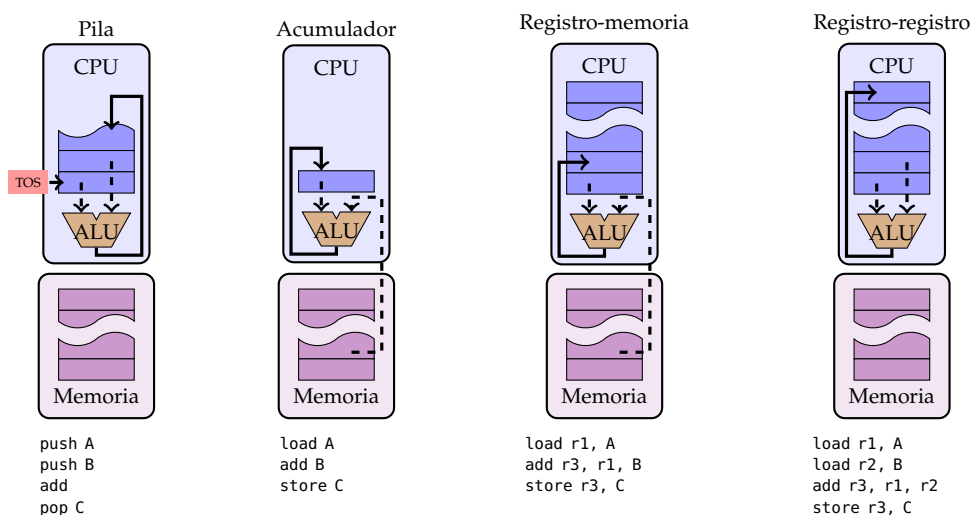
Figura 1.3: Tipos de modelo de máquina
