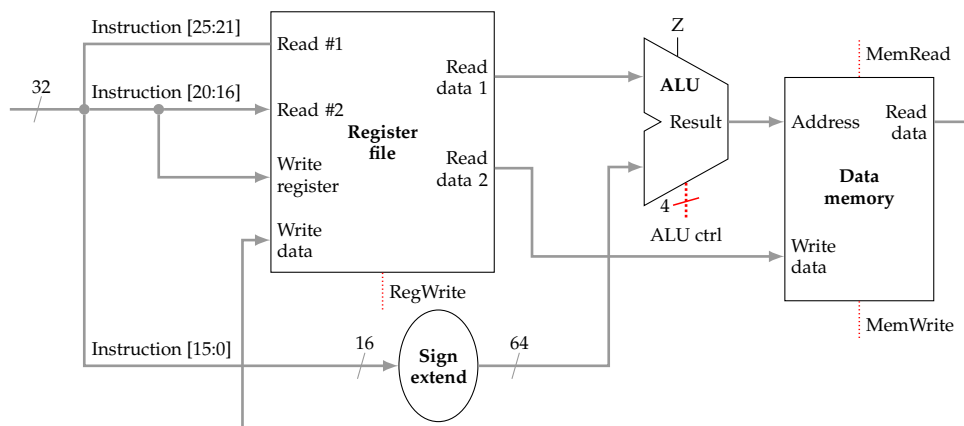
Figura 2.11: Ejecución de instrucciones de carga y almacenamiento
