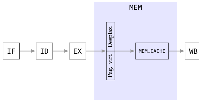
Figura 3.55: Caché indexada y etiquetada virtualmente (V/V)
