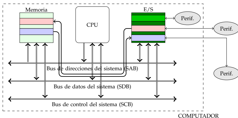
Figura 4.1: Operaciones de entrada y salida dentro del computador von Neumann
