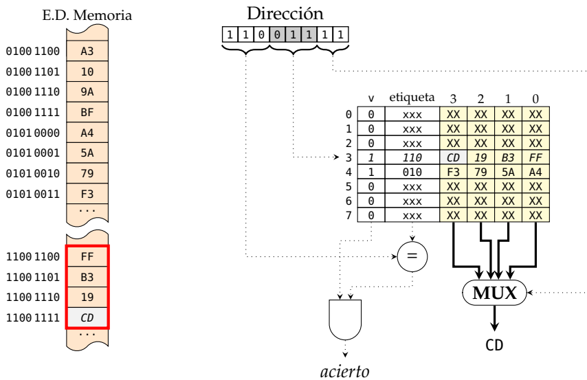
Figura 3.16: Correspondencia directa: reemplazo del bloque en la línea 3 y la caché sirve el byte solicitado
