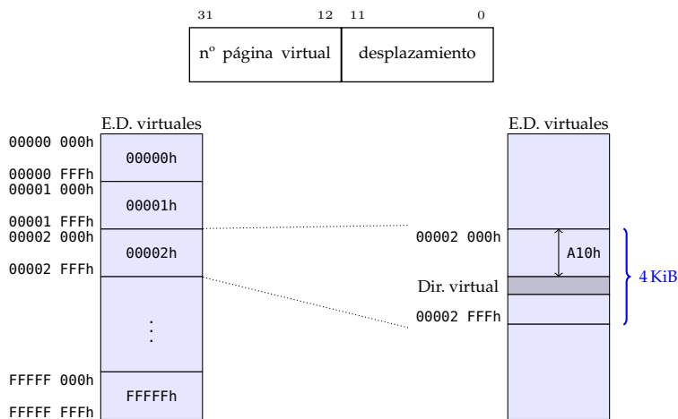
Figura 3.41: Traducción por bloques de las direcciones virtuales a direcciones físicas
