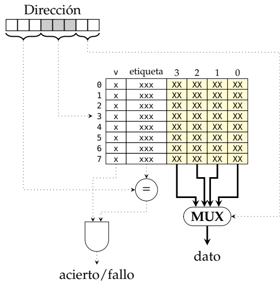
Figura 3.7: Estructura de una caché con correspondencia directa
