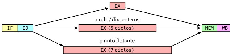
Figura 2.25: Introducción de operaciones multiciclo de enteros y punto flotante
