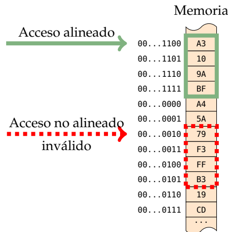
Figura 2.4: Accesos alineados y no alineados a palabras en memoria
