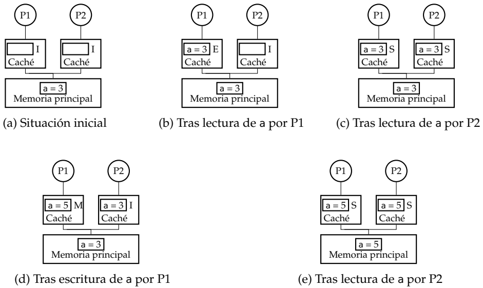
Figura 3.36: Ejemplo de funcionamiento del protocolo MESI
