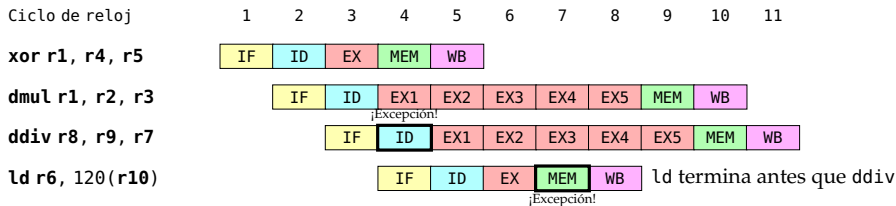
Figura 2.31: La terminación fuera de orden puede ocasionar excepciones no precisas
