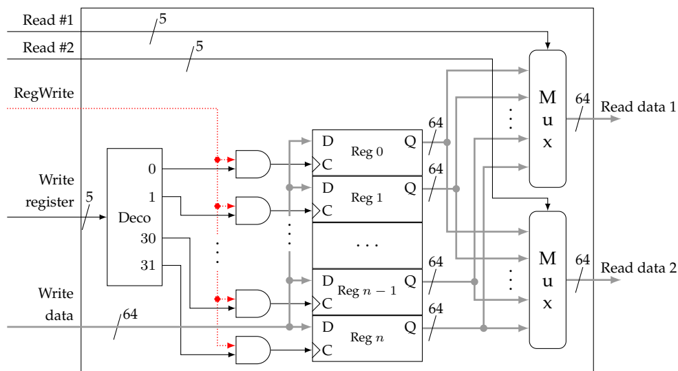
Figura 2.6: Posible implementación del fichero de registros
