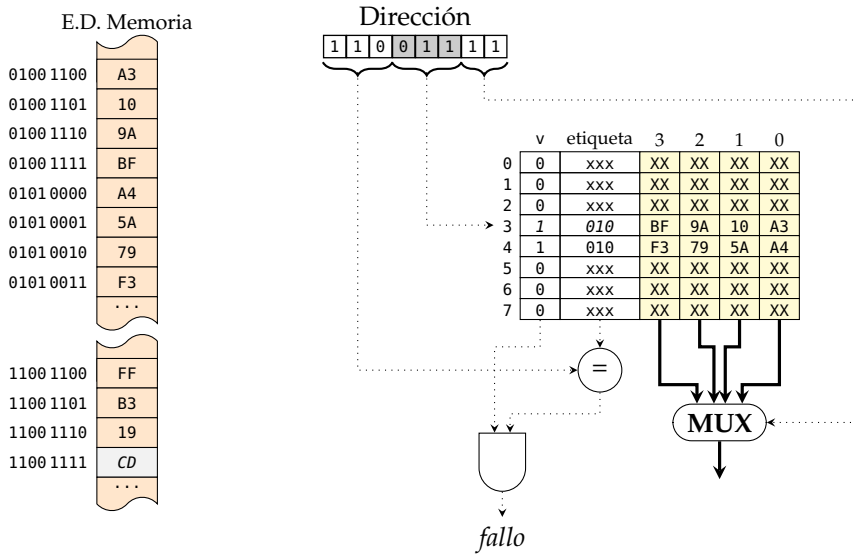
Figura 3.15: Correspondencia directa: petición de lectura de un byte sobre la dirección CFh, que produce un fallo de caché
