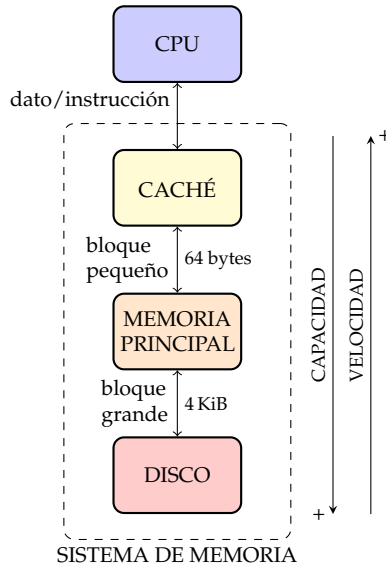
Figura 3.3: Jerarquía de memoria de tres niveles
