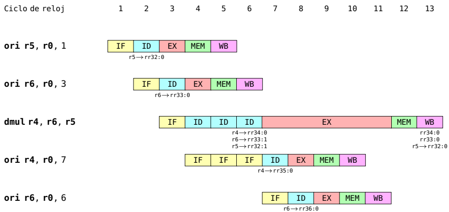
Figura 2.46: Ejecución con renombrado de registros a nivel hardware
