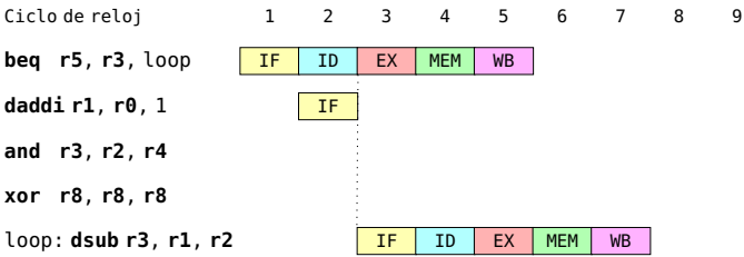
Figura 2.48: Detención por riesgo de control con evaluación agresiva de saltos suponiendo que el salto se toma
