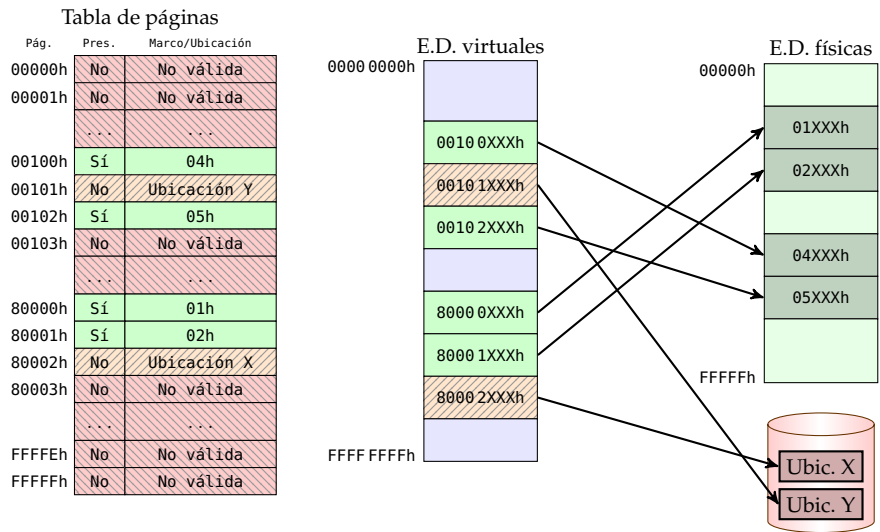
Figura 3.44: La tabla de páginas de una tarea
