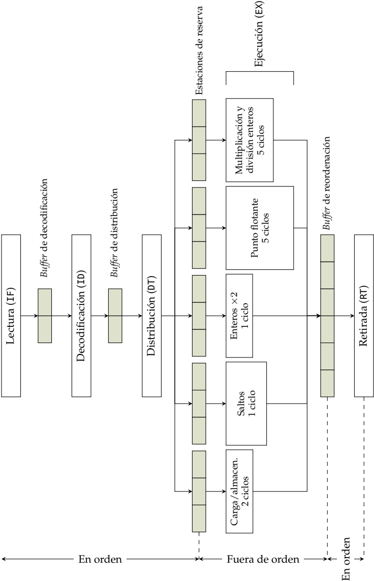
Figura 2.55: Organización de una CPU superescalar
