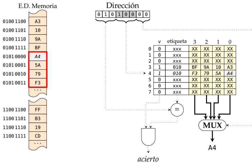
Figura 3.13: Correspondencia directa: se carga la línea 4 y la caché sirve el byte solicitado
