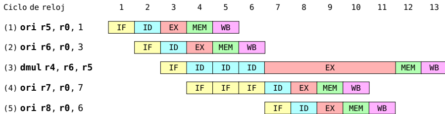
Figura 2.45: Ejecución sin reciclaje de registros
