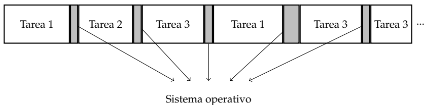
Figura 2.62: Cronograma de ejecución del SO y tres tareas
