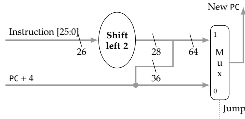
Figura 2.15: Ejecución de la instrucción de salto incondicional j
