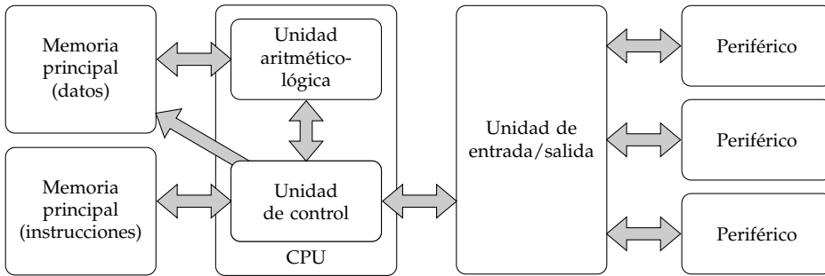
Figura 2.1: Arquitectura Harvard
