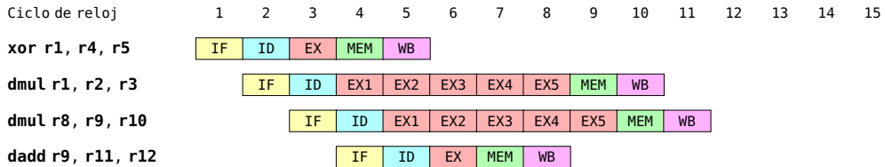
Figura 2.29: Ejecución de operaciones multiciclo segmentadas
