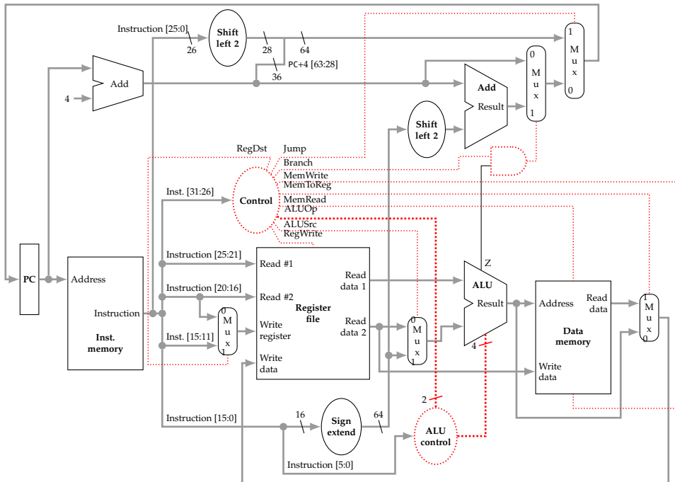
Figura B.2: Camino de datos para la ejecución de instrucciones de tipo R, acceso a memoria, salto condicional beq y salto incondicional j con la lógica de control
