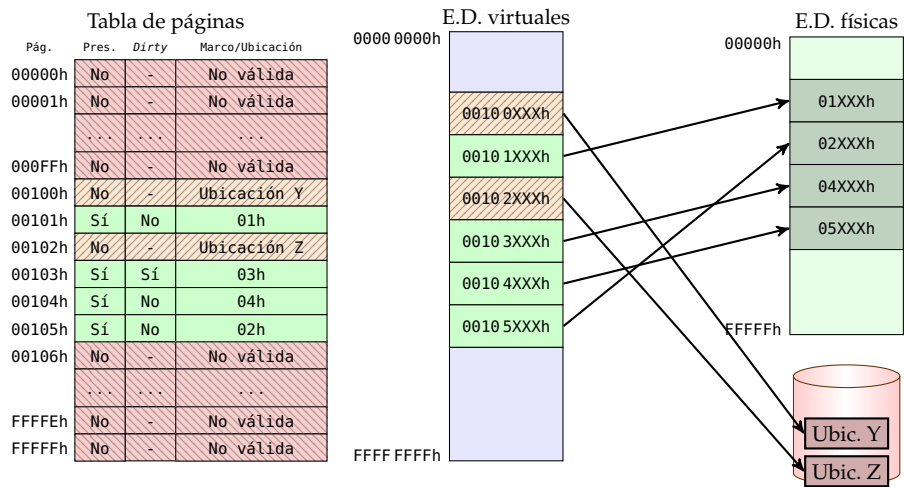
Figura 3.52: Carga desde el disco de la página 00105h
