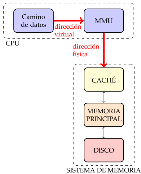
Figura 3.38: Traducción de direcciones virtuales a direcciones físicas
