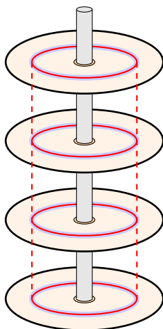
Figura 4.14: Definición del cilindro en un disco duro
