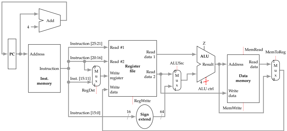
Figura 2.12: Camino de datos para la ejecución de instrucciones de tipo R y de carga/almacenamiento
