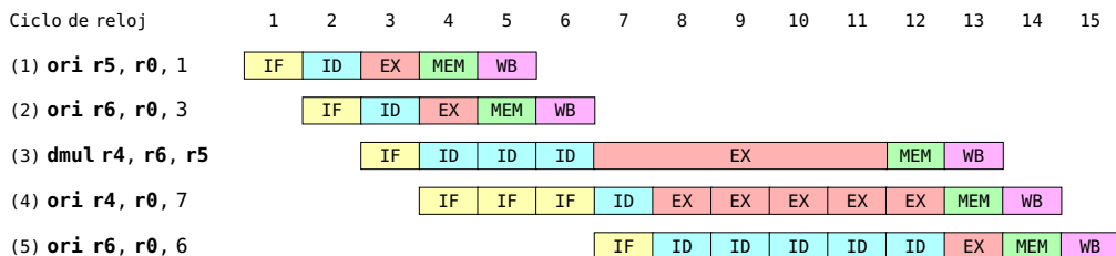
Figura 2.43: Ejecución con reciclaje de registros
