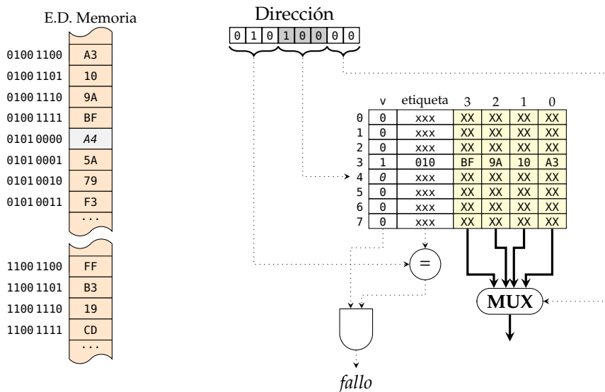
Figura 3.12: Correspondencia directa: petición de lectura de un byte sobre la dirección 50h, que produce un fallo de caché
