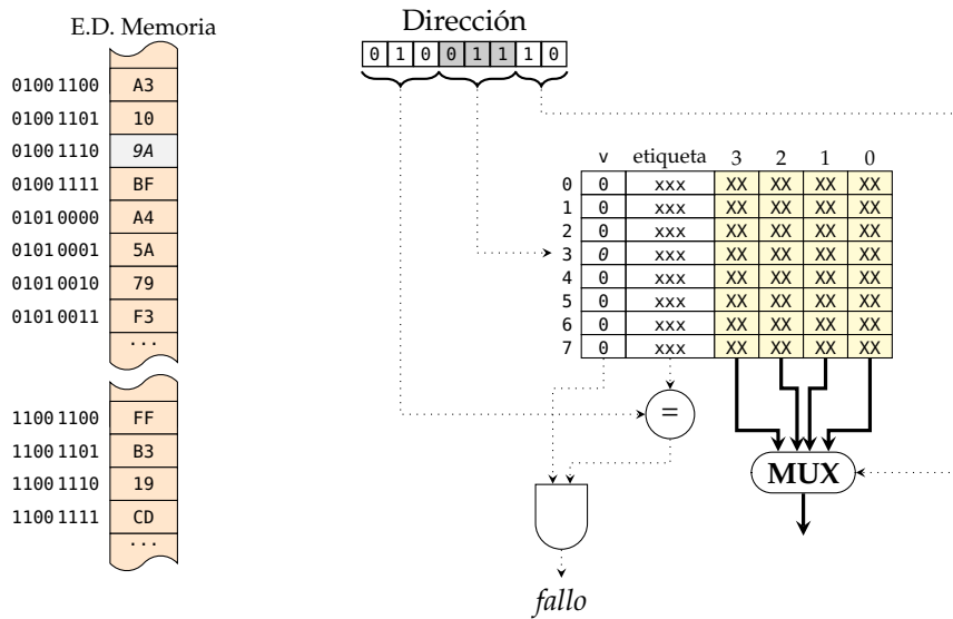
Figura 3.9: Correspondencia directa: petición de lectura de un byte sobre la dirección 4Eh, que produce un fallo de caché
