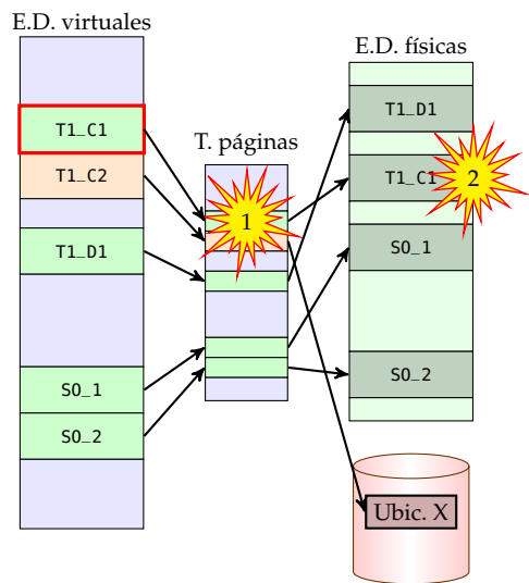
Figura 3.53: Acceso a memoria empleando paginación sin TLB
