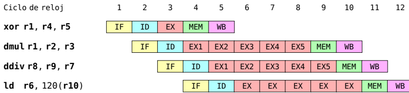
Figura 2.32: Las excepciones precisas requieren terminación en orden
