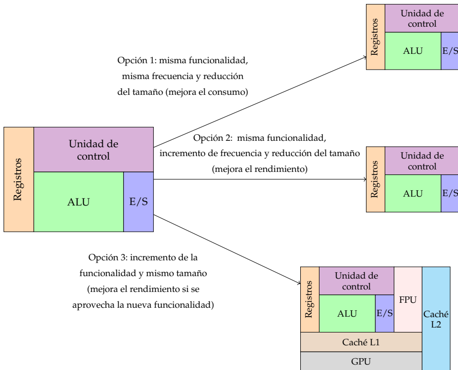
Figura 2.59: Posibilidades de mejora tras reducir la tecnología de fabricación
