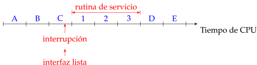
Figura 4.5: Ejecución de un programa con una interrupción
