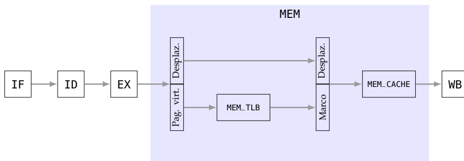
Figura 3.54: Segmentación en el acceso al TLB y a la caché
