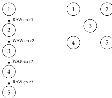
Figura 2.54: Ejemplos de paralelismo a nivel de instrucción
