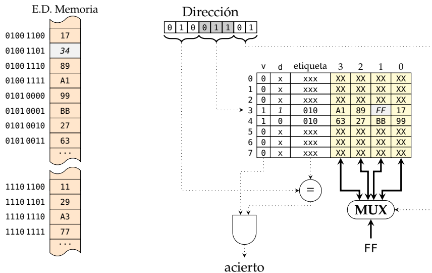
Figura 3.27: Funcionamiento de la estrategia de escritura write-back : petición de escritura de un byte sobre la dirección 4Dh; acierto, el bloque se marca como sucio
