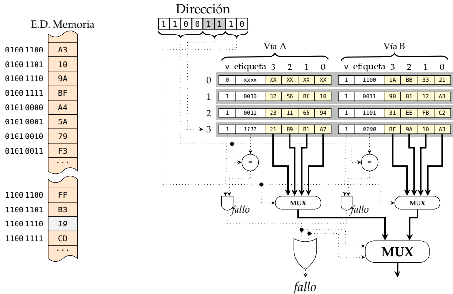
Figura 3.24: Correspondencia asociativa por conjuntos: petición de lectura de un byte sobre la dirección CEh, que produce un fallo de caché
