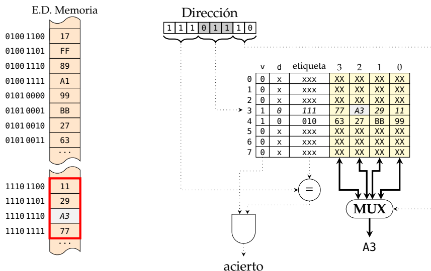
Figura 3.30: Funcionamiento de la estrategia de escritura write-back : reemplazo del bloque en la línea 3 y la caché sirve el byte solicitado
