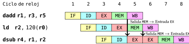
Figura 2.40: Activación de dos rutas de reenvío durante la ejecución de una instrucción
