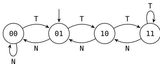
Figura 2.51: Máquina de estados y memoria de saltos de un predictor de 2 bits
