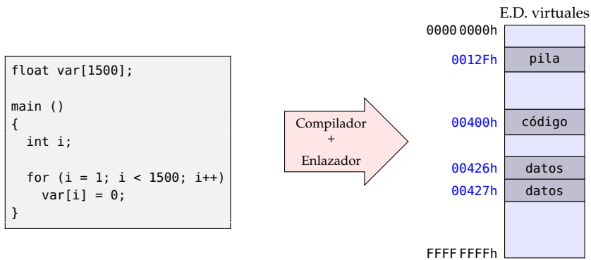
Figura 3.46: Ejemplo de ubicación del código y datos de un programa dentro del espacio de direcciones virtuales de una tarea
