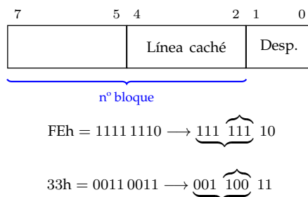
Figura 3.5: Ejemplo de obtención del número de bloque de memoria y línea de caché con correspondencia directa
