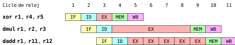
Figura 2.27: Ejemplo de detención WAW ocasionada por unidades de ejecución multiciclo
