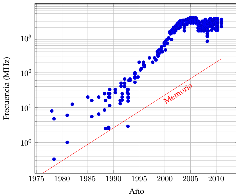
Figura 3.1: Evolución en velocidad de la CPU y la memoria
