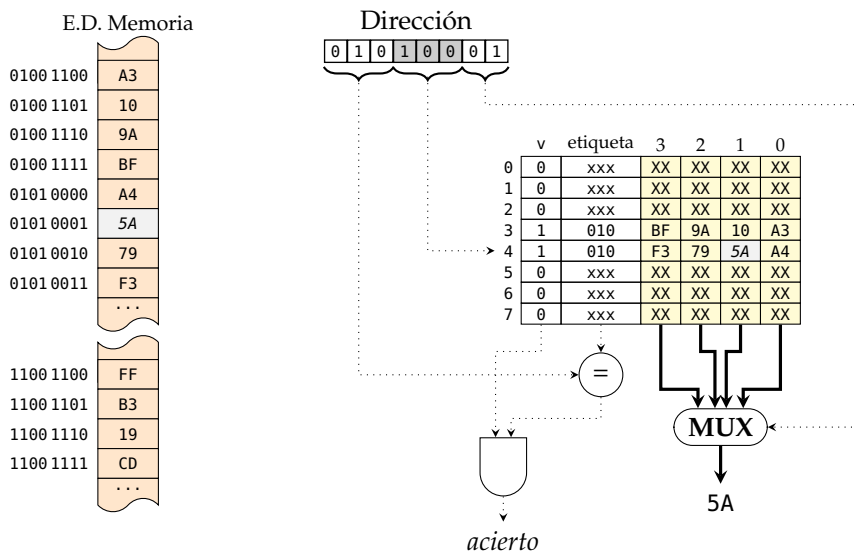
Figura 3.14: Correspondencia directa: petición de lectura de un byte sobre la dirección 51h, que produce un acierto de caché
