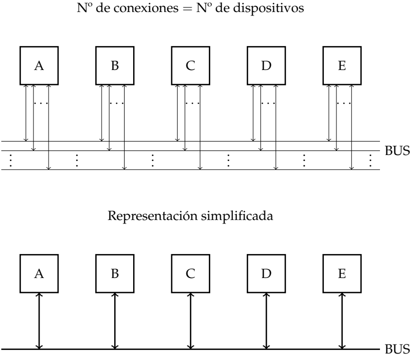
Figura 4.9: Conexión de los dispositivos mediante un bus
