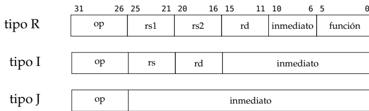
Figura 2.5: Codificación de instrucciones en MIPS64
