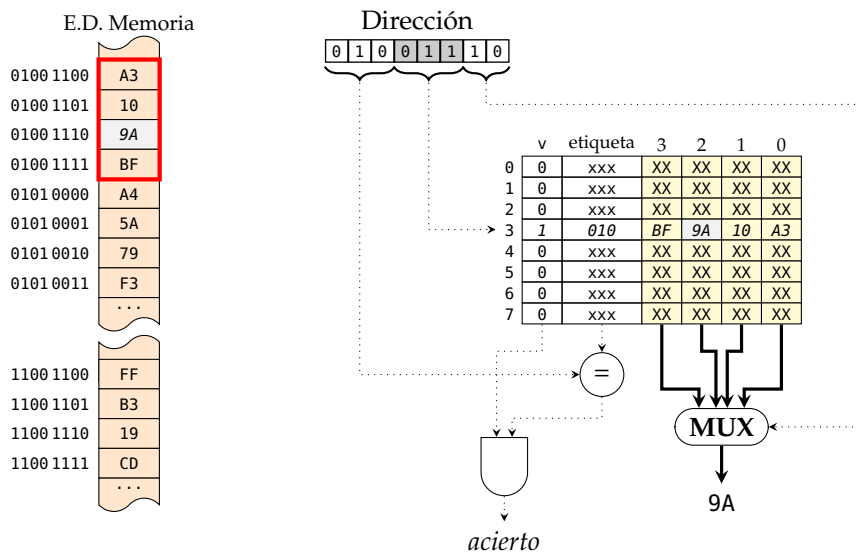
Figura 3.10: Correspondencia directa: se carga la línea 3 y la caché sirve el byte solicitado
