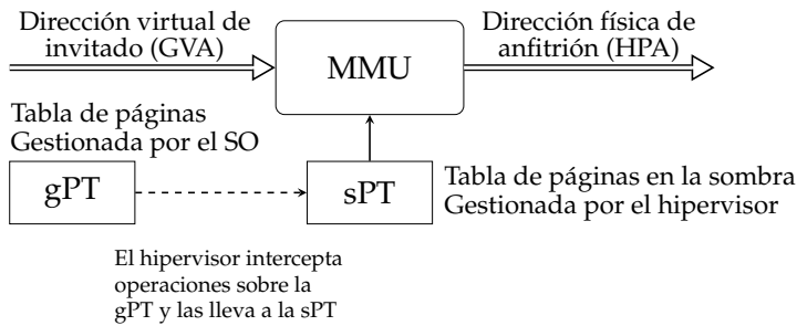
Figura 3.60: Traducción empleando tablas de páginas en la sombra
