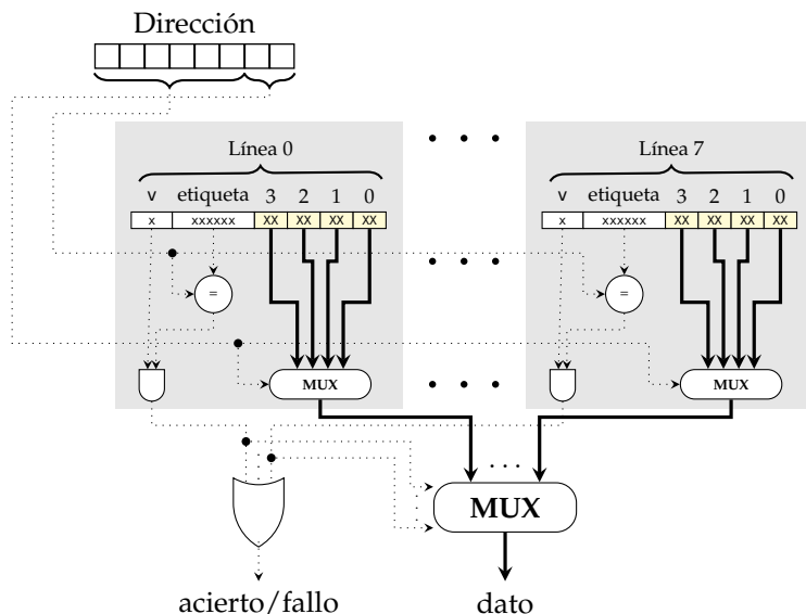
Figura 3.18: Estructura de una caché con correspondencia totalmente asociativa
