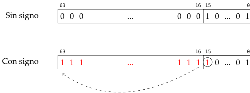
Figura 2.3: Carga de la media palabra 90BDh en un registro sin signo ( zero-extended ) y con signo ( sign-extended )
