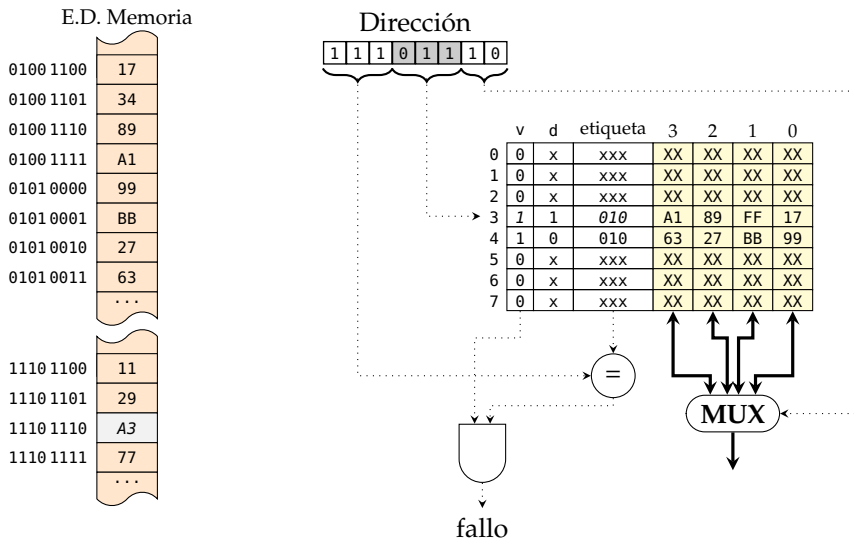
Figura 3.28: Funcionamiento de la estrategia de escritura write-back : petición de lectura de un byte sobre la dirección EEh, que origina un fallo de caché
