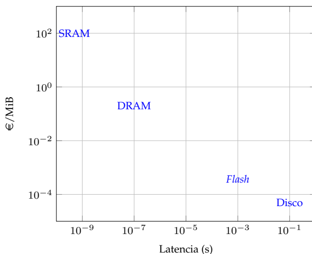
Figura 3.2: Relación coste y velocidad de las tecnologías de memoria
