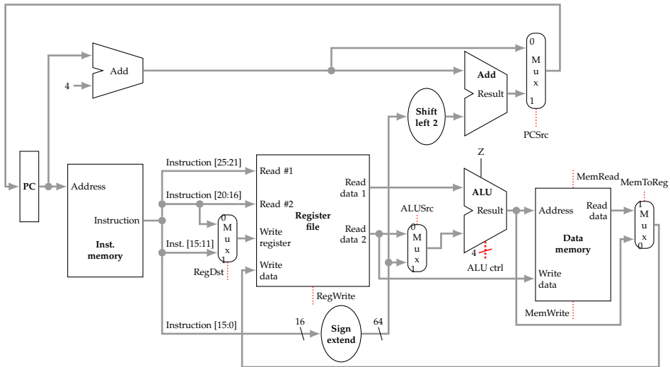
Figura 2.14: Camino de datos para la ejecución de instrucciones de tipo R, carga/almacenamiento y salto condicional beq
