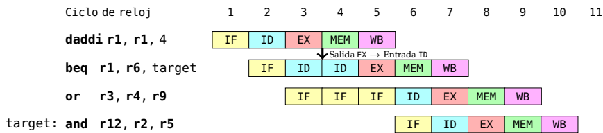
Figura 2.49: Nueva ruta de reenvío Salida EX → Entrada ID con evaluación agresiva de saltos. El salto no se toma.
