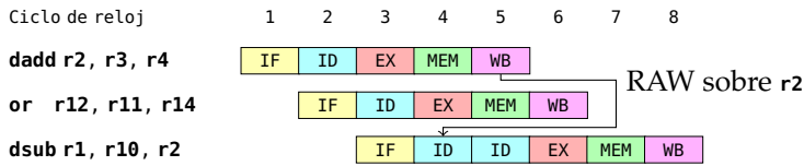
Figura 2.33: Efecto de la reordenación de instrucciones
