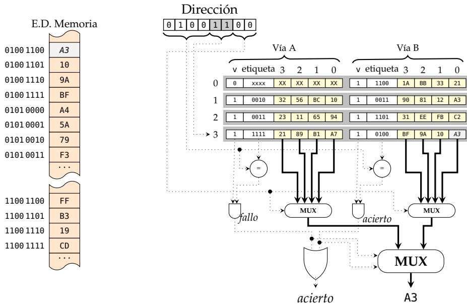
Figura 3.23: Correspondencia asociativa por conjuntos: petición de lectura de un byte sobre la dirección 4Ch, que produce un acierto de caché
