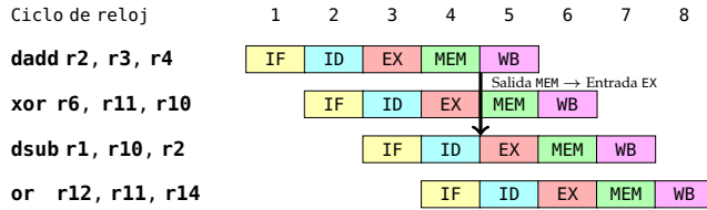
Figura 2.36: Ruta de reenvío Salida MEM → Entrada EX
