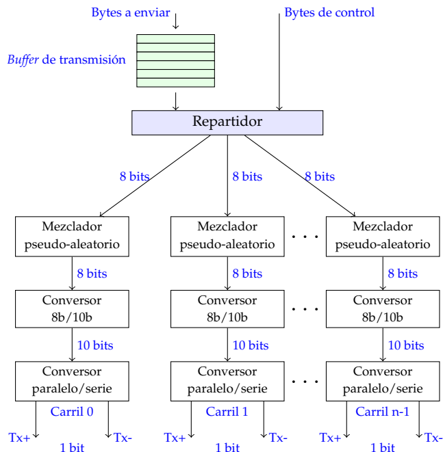
Figura 4.11: Procesamiento del paquete a enviar por un dispositivo PCI Express
