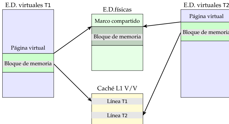
Figura 3.56: El problema de los sinónimos en las cachés virtuales
