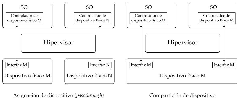
Figura 4.17: Virtualización de dispositivos por hardware
