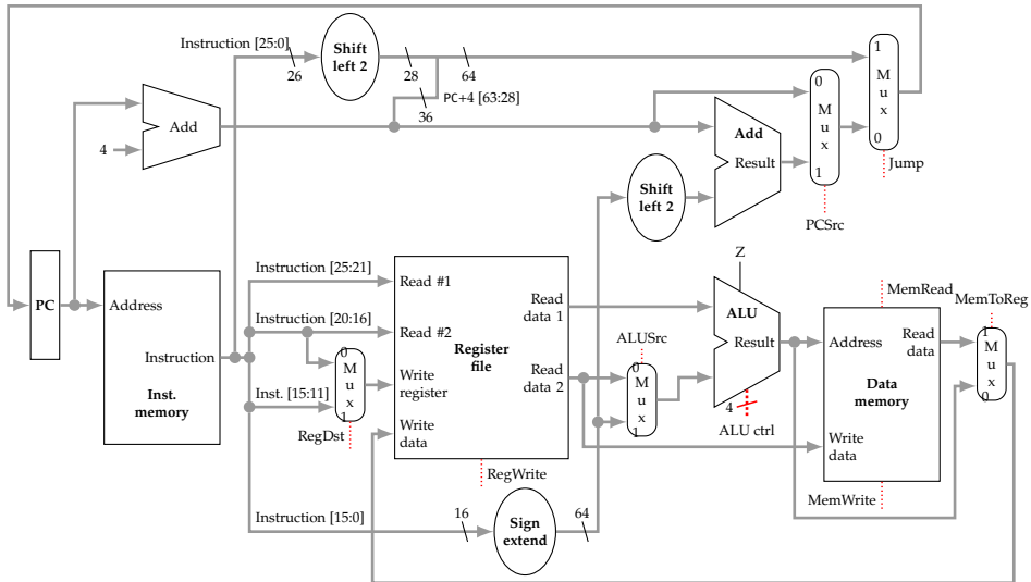
Figura 2.16: Camino de datos para la ejecución de instrucciones de tipo R, acceso a memoria, salto condicional beq y salto incondicional j
