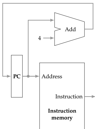
Figura 2.8: Búsqueda de la instrucción a ejecutar e incremento del PC
