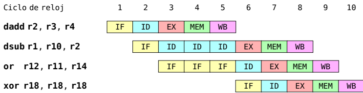
Figura 2.22: Ejecución segmentada con una detención por dependencia de datos
