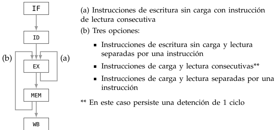
Figura 2.41: Resumen de las rutas de reenvío
