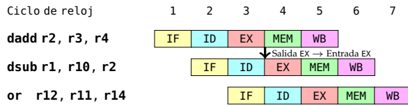
Figura 2.34: Ejecución con la ruta de reenvío Salida EX → Entrada EX
