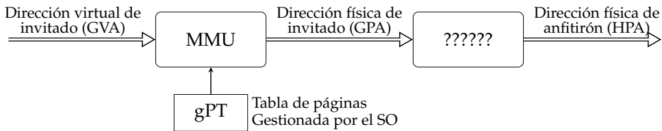
Figura 3.59: Traducción entre los tres espacios de direcciones
