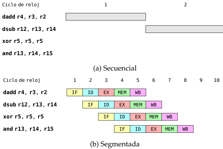
Figura 2.18: Ejecución de instrucciones de forma secuencial y segmentada
