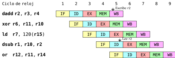
Figura 2.37: La ruta de reenvío Salida WB → Entrada EX no es necesaria
