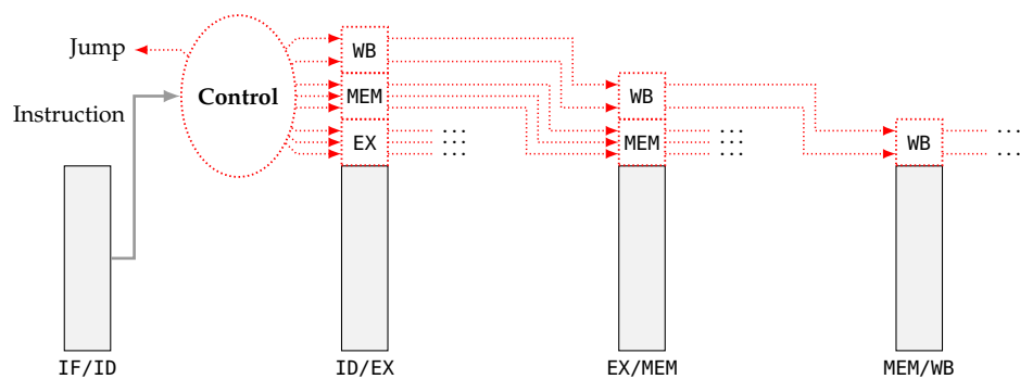
Figura B.4: Propagación de las señales de control en el camino de datos segmentado
