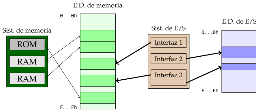
Figura 4.2: Ejemplo de ubicación en los espacios de direcciones
