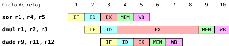
Figura 2.26: Mejoras de rendimiento empleando varias unidades de ejecución
