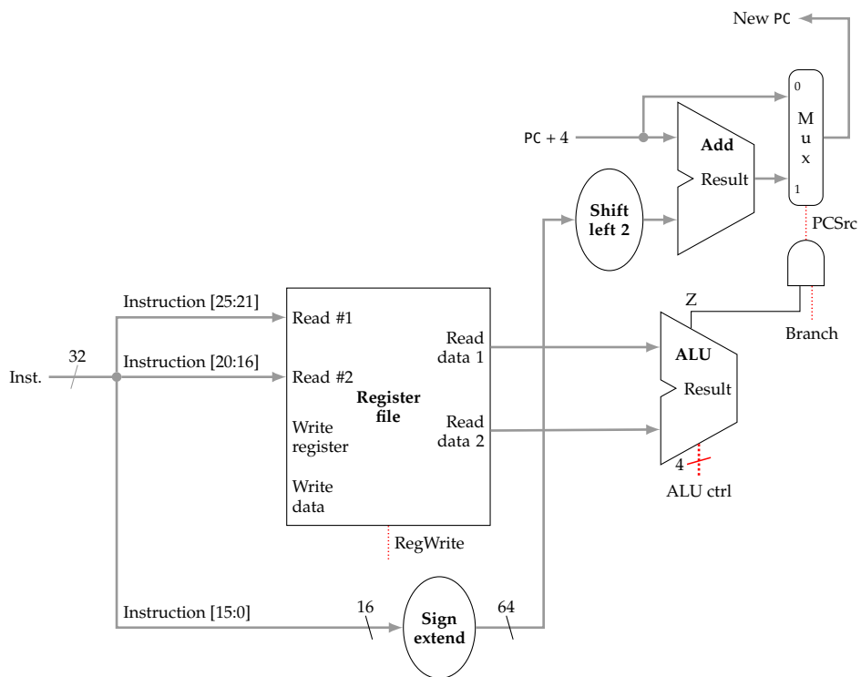
Figura 2.13: Ejecución de la instrucción de salto condicional beq
