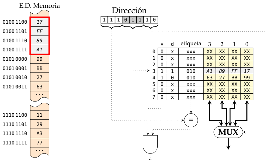
Figura 3.29: Funcionamiento de la estrategia de escritura write-back : actualización del bloque sucio en el espacio de direcciones de memoria
