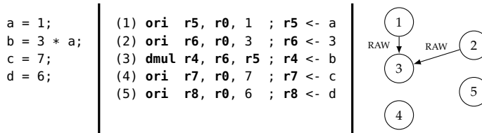
Figura 2.44: Eliminación de dependencias WAR y WAW evitando el reciclaje de registros
