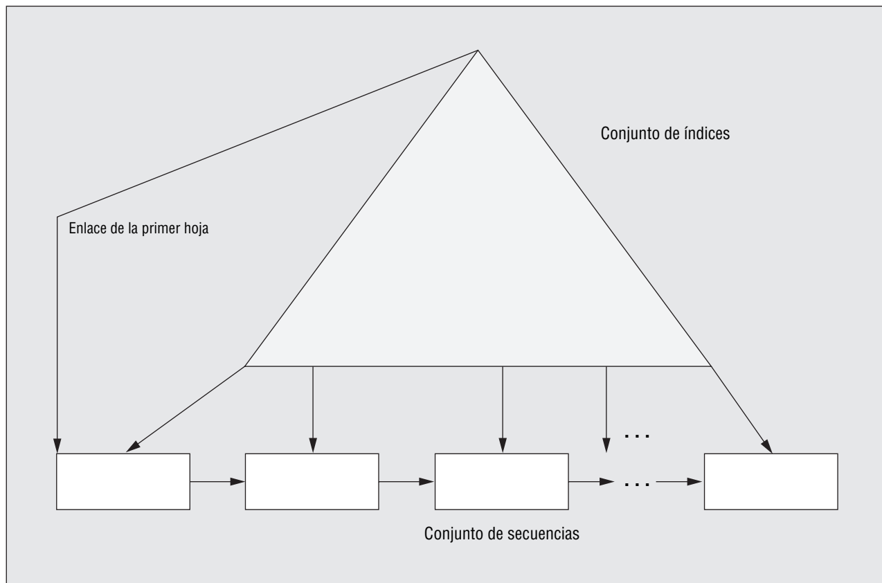
FIGURA 8.14 Estructura B+Tree
