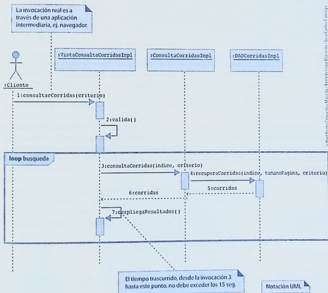
» Figura 4-5. Ejemplo de una vista de comportamiento
