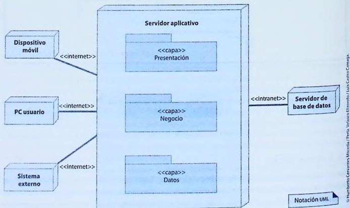
» Figura 4-6. Ejemplo de una vista física
