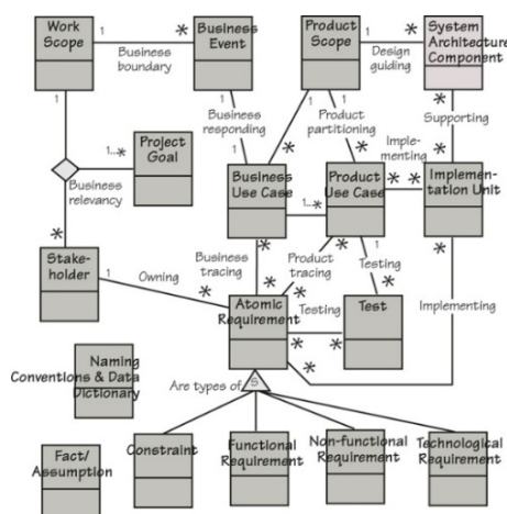
Figura 16. Volere model [49]
