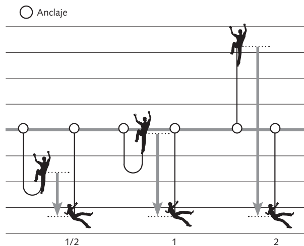
GRÁFICO 6.5 Sistemas de anclaje. Factor de caída: 1/2, 1 y 2. Trabajar máximo con factor de caída 1.
