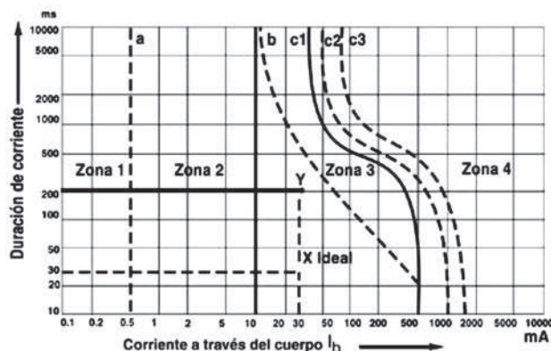
GRÁFICO 1.9 Corriente a través del cuerpo. Efectos fisiológicos.
