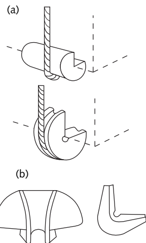
GRÁFICO 3.11 Cantoneras para cuerdas (tomado de S.T. XII.12 INHST).
