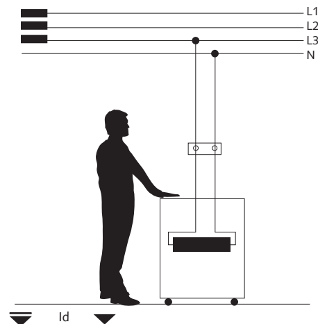
GRÁFICO 1.7 Contacto eléctrico indirecto.
