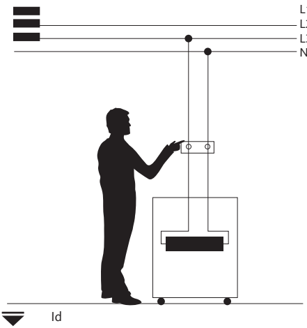
GRÁFICO 1.5 Contacto eléctrico directo.
