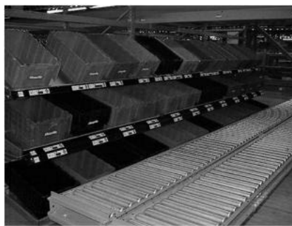
Fotografía 10. Estanterías móviles.
