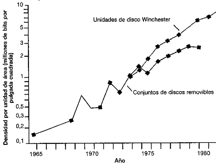
Figura 1.5 Impacto de la arquitectura Winchester sobre las tecnologías ya establecidas en la densidad de grabación de las unidades de disco de 14 pulgadas
