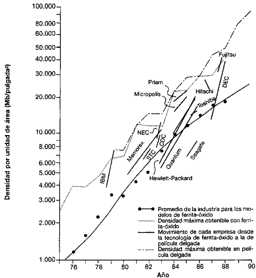
Figura 6.1 Puntos en los cuales la tecnología de película delgada fue adoptada por los fabricantes líderes, en relación con las capacidades de la tecnología de ferrita-óxido en el momento de efectuar el cambio
