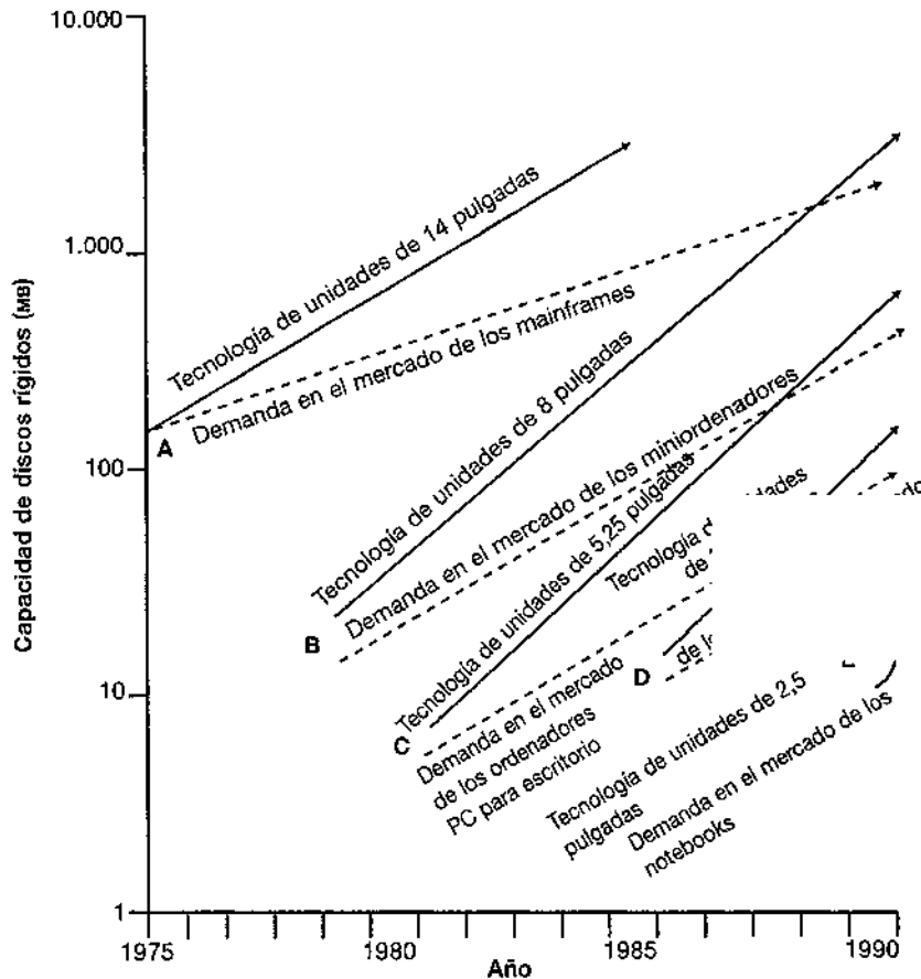
Figura 1.7 Trayectorias intersecantes de capacidad demandada versus capacidad suministrada en unidades de discos rígidos
