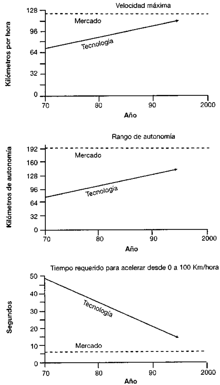
Figura 9.1 El automóvil eléctrico
