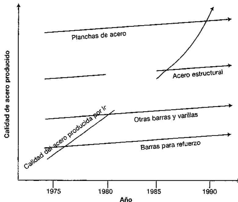
Figura 4.3: El progreso de la tecnología de punta de los minilaminadores
