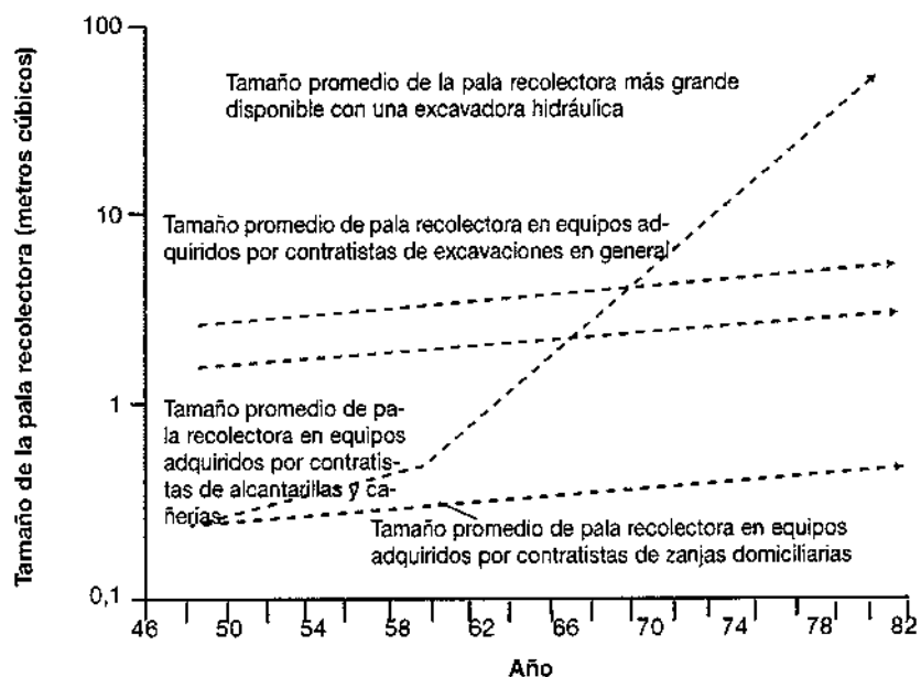
Figura 3.3 Impacto abrupto de la tecnología hidráulica de punta en el mercado de los excavadores mecánicos.
