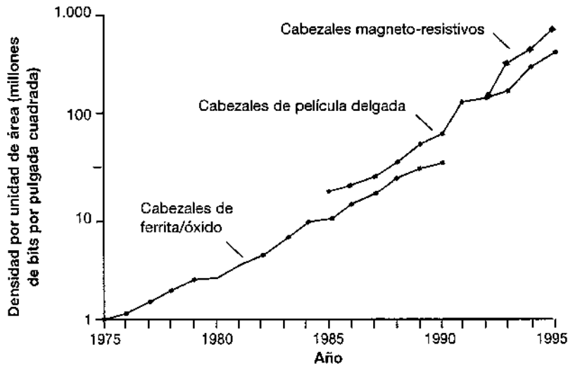
Figura 1.4 Impacto de las nuevas tecnologías de cabezales de lectura-escritura sobre las tecnologías ya establecidas en el mejoramiento de la densidad de grabación
