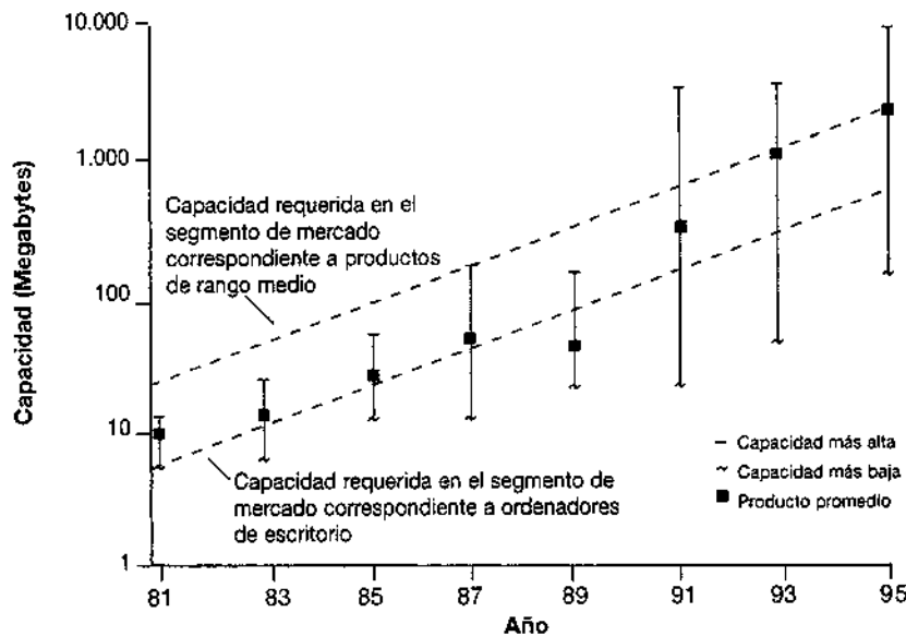
Figura 4.1 Migración mercado arriba de las unidades de disco de Seagate
