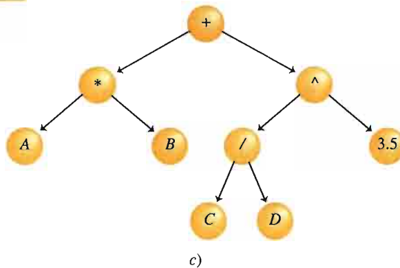
FIGURA 6.20 Ejemplo de un árbol binario
