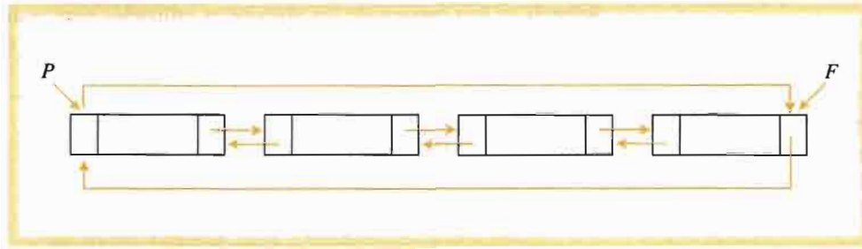
FIGURA 5.24 Listas doblamente ligadas circular.
