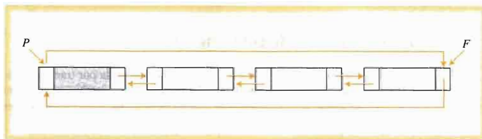
FIGURA 5.25 Listas doblamente ligadas con nodo de cabecera.
